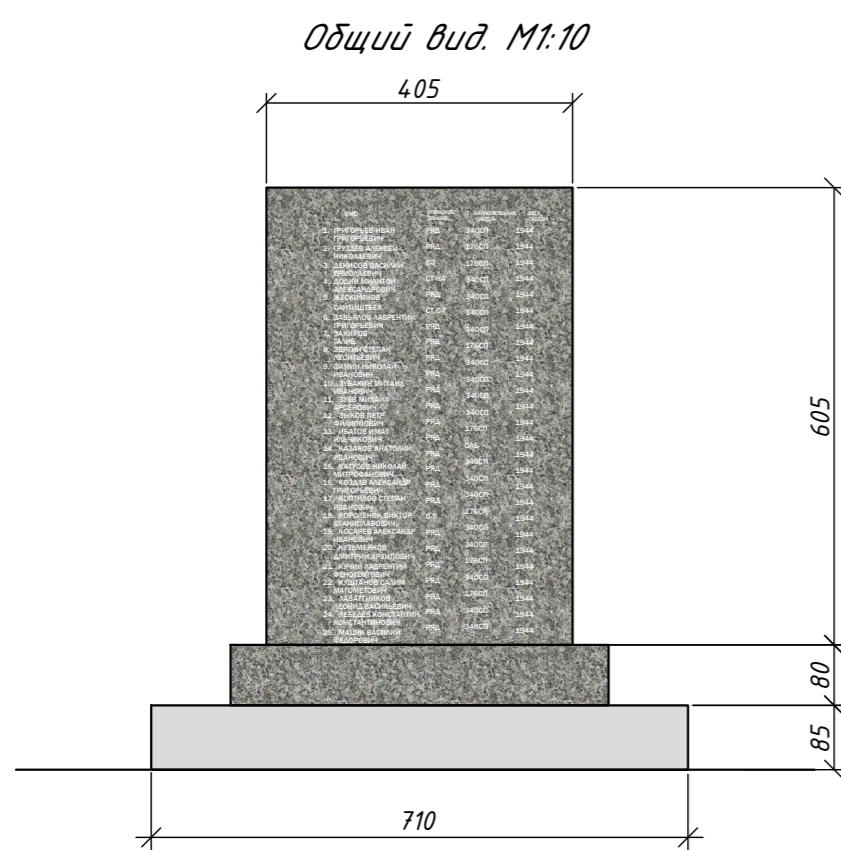
Мемориальная плита МП 12. Тип 2.
