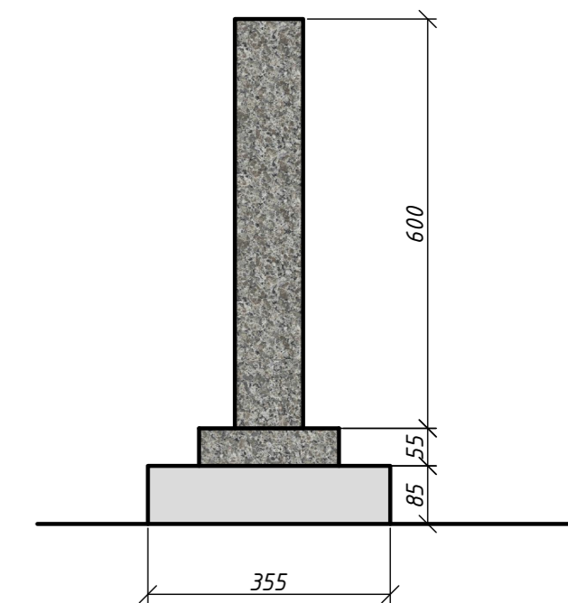
Вид сбоку. М1:10
