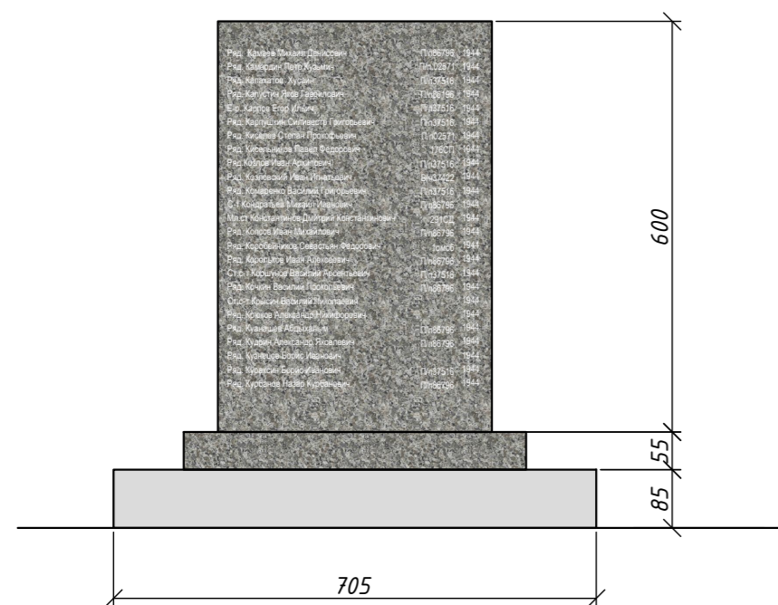
Общий вид. М1:10
