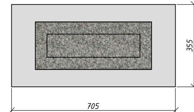
Вид сверху. М1:10
