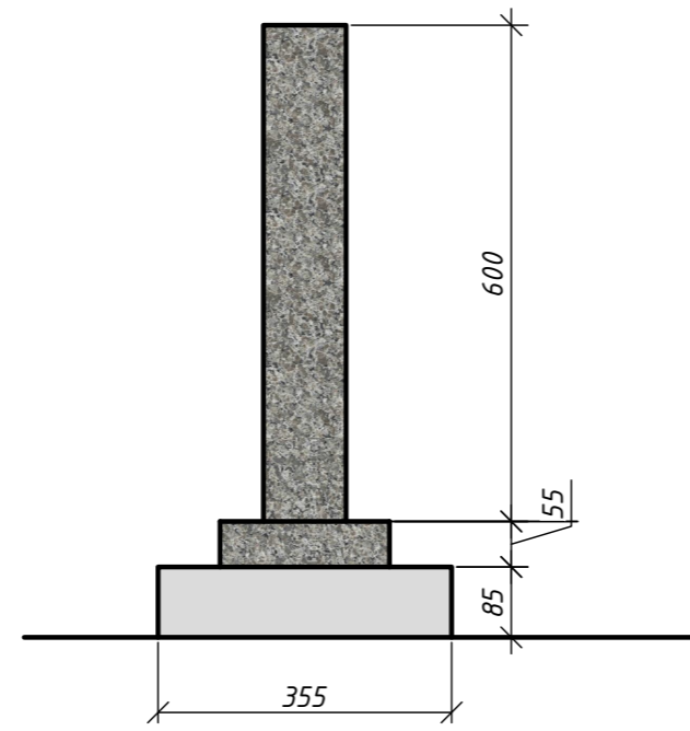
Вид сбоку. М1:10
