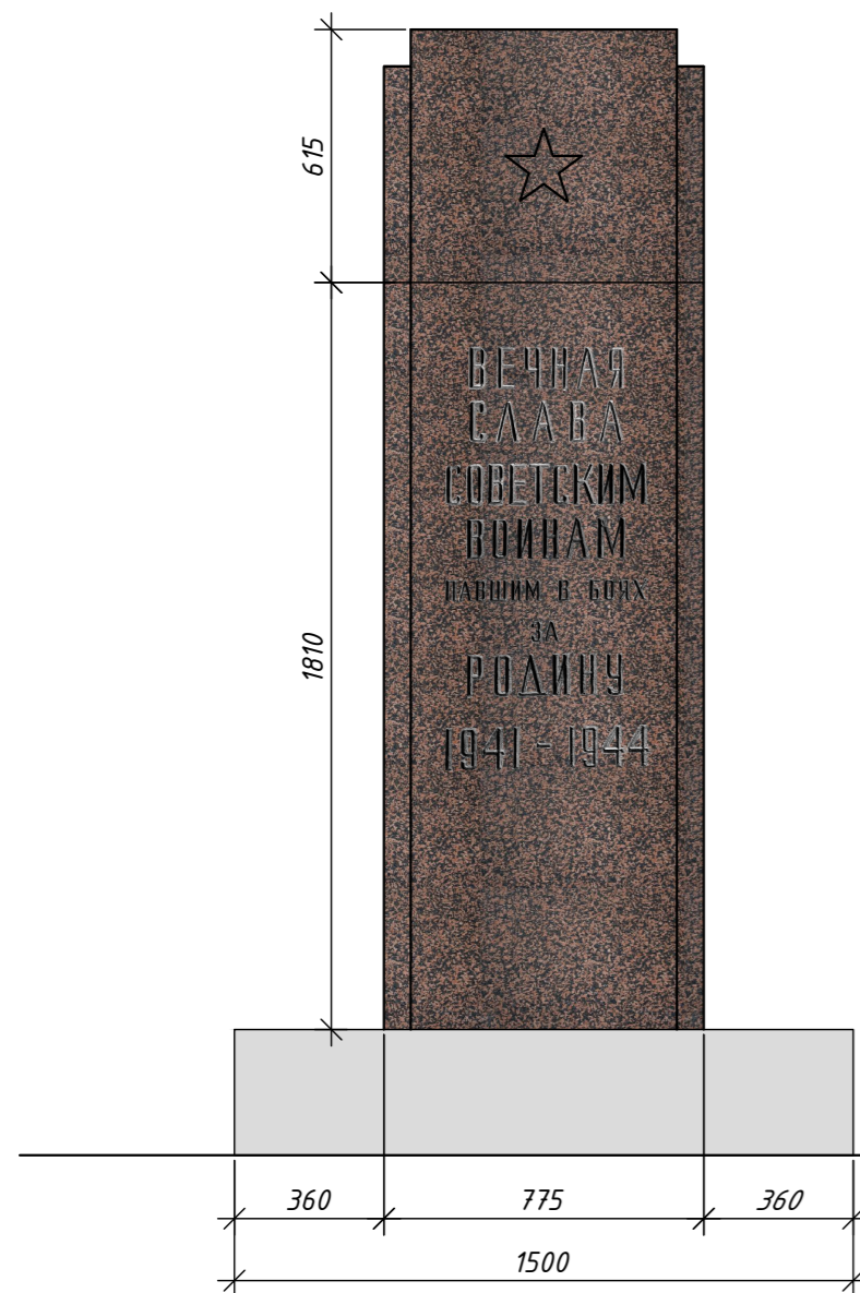
Общий вид. М1:20
