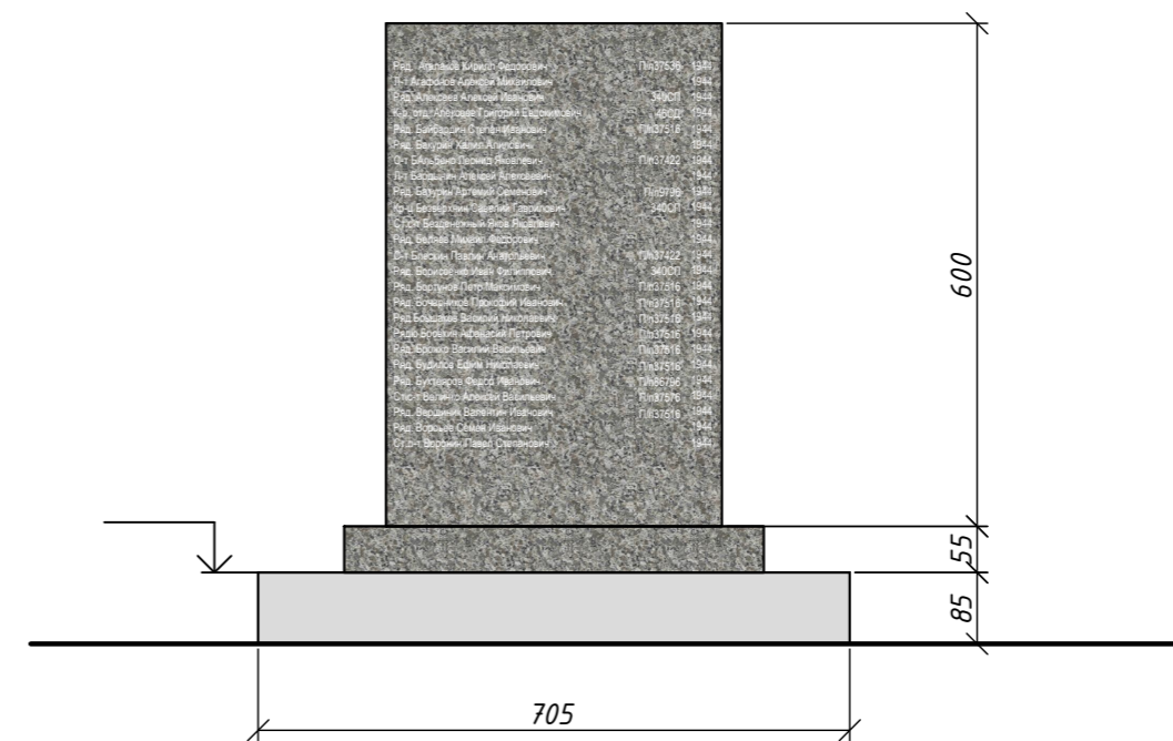
Общий вид. М1:10
