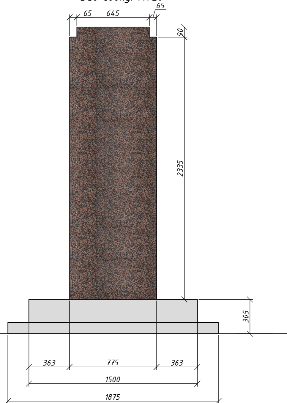
Вид сбоку. М1:20
