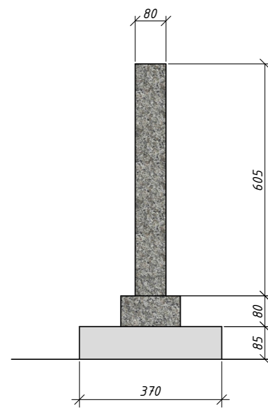
Вид сбоку. М1:10
