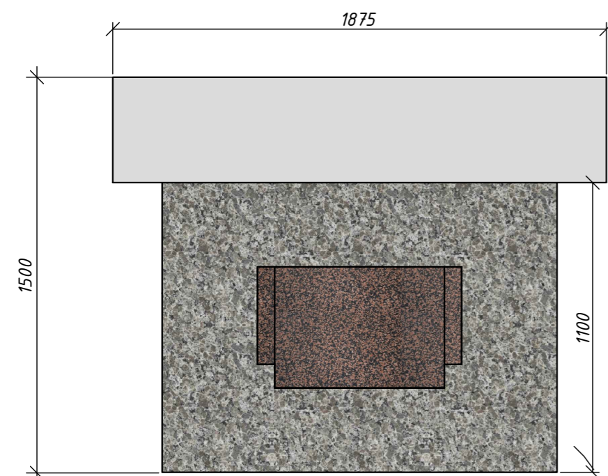
Вид сверху. М1:20
