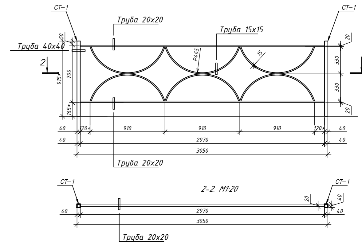
Типовая секция SK2. Общий вид. М1:20
