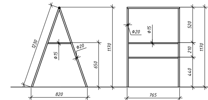
Подставка под венки. Вид сбоку. М1:20 Подставка под венки. Вид спереди. М1:20
