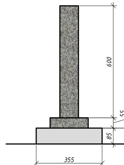
Вид сбоку. М1:10
