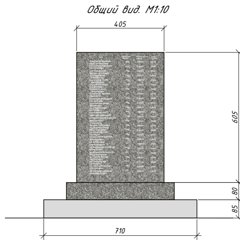
Мемориальная плита МП 10. Тип 2.
