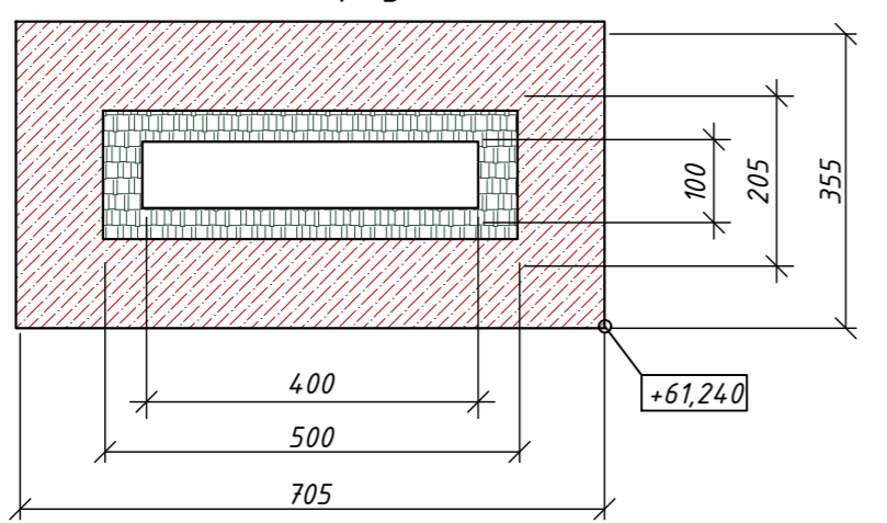
Вид сверху М1:10
