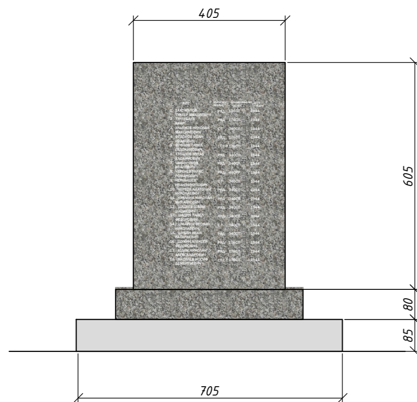
Общий вид. М1:10
