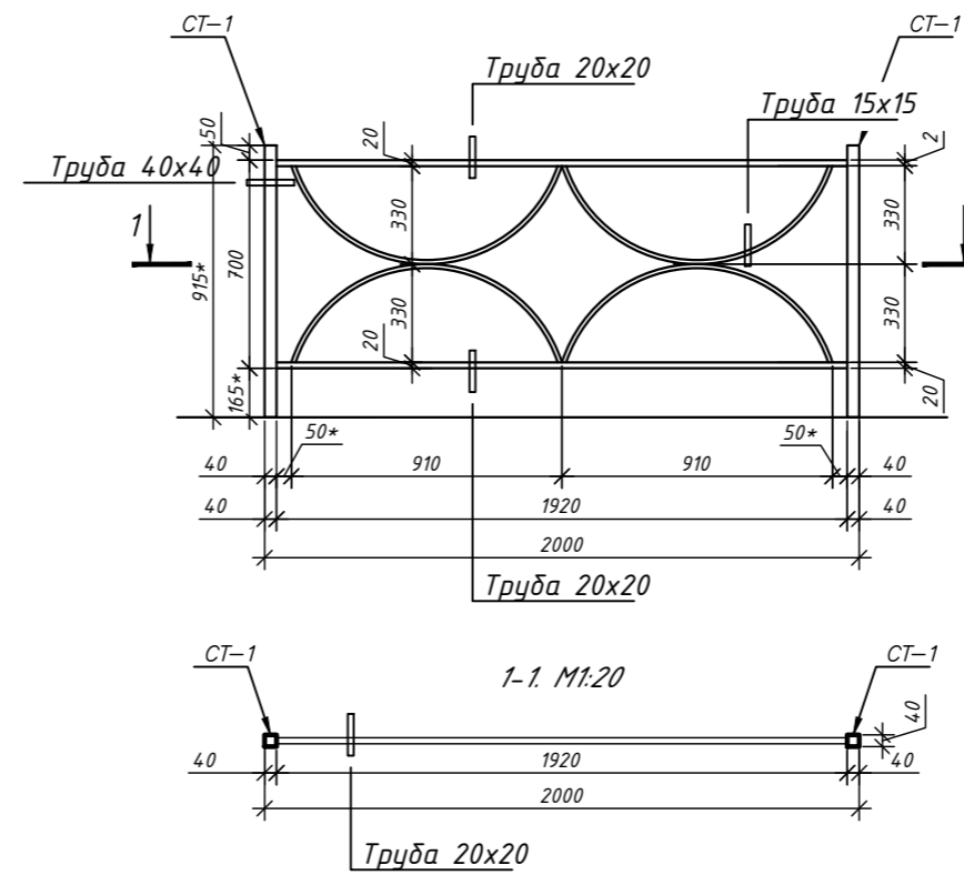
Ведомость металлического ограждения
