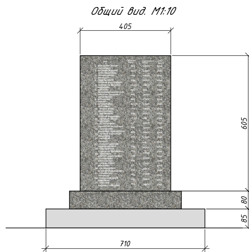
Мемориальная плита МП 11. Тип 2.
