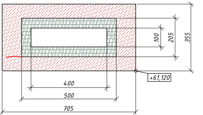
Вид сверху М1:10
