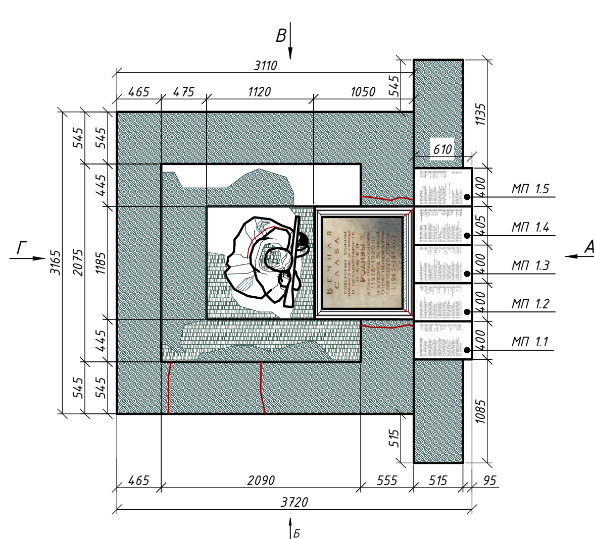
Постамент скульптуры воина. Вид сверху. М 1:40
