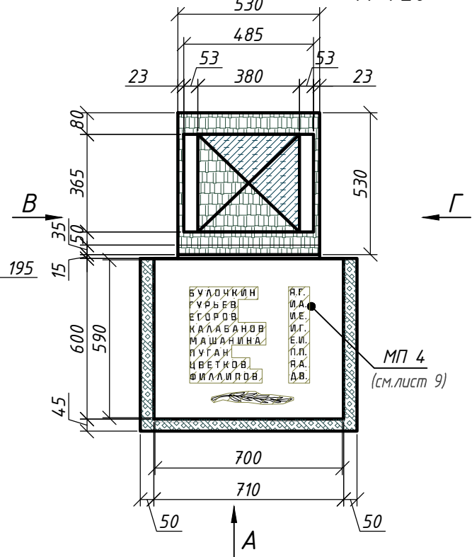
Стела 2. Вид сверху. М 1:20
