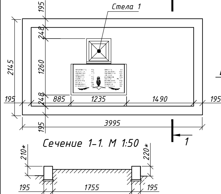
План-схема братской могилы Тип 1.1. М 1:50
