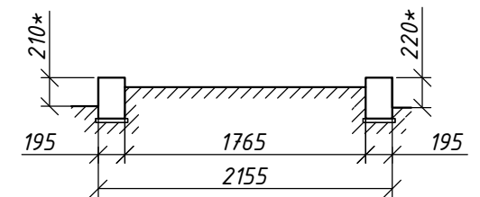
Братская могила Тип 2.1-2.2. Сечение 1-1. М
