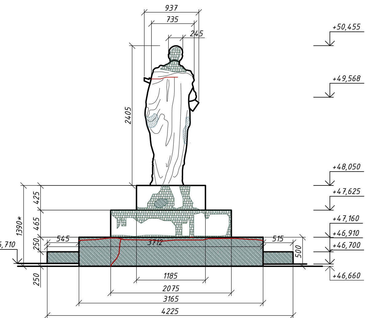
Скульптура воина на постаменте. Вид В. М 1:40
