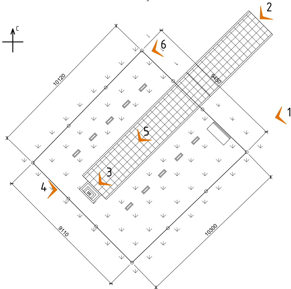
План участка
