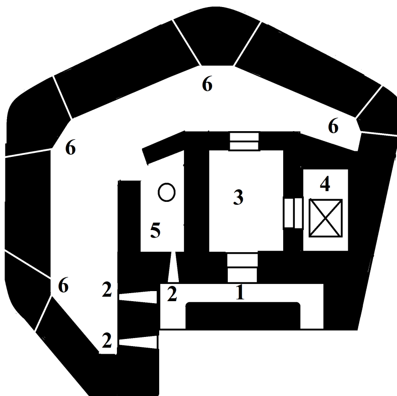
ДОТ № 975. План-схема верхнего этажа:
