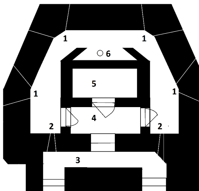
ДОТ № 951. План-схема верхнего этажа:
