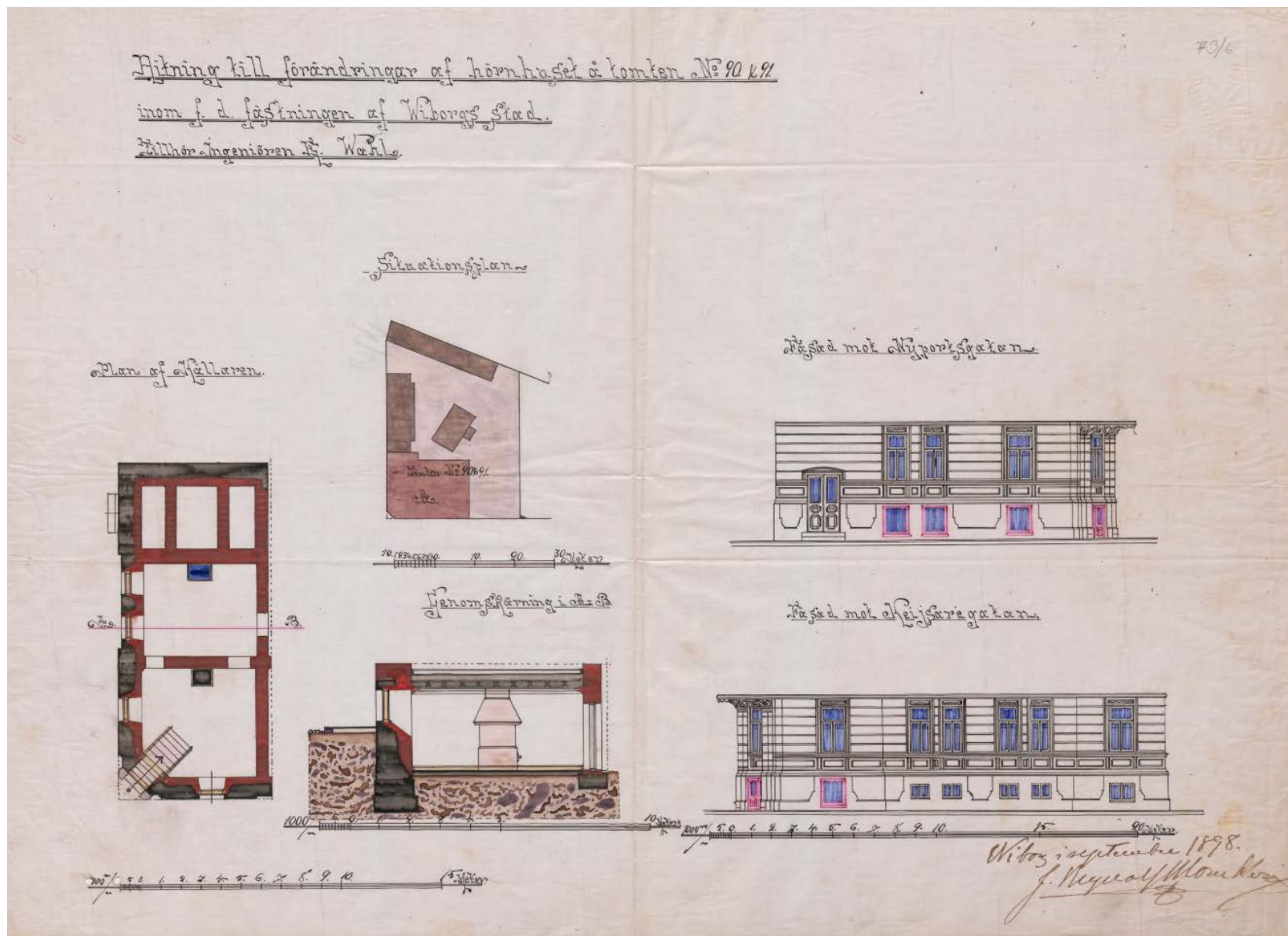
Илл. 8. Чертеж хозяйственного дома. Владение наследников Шабарина. 1898 г. // по Акту ГИКЭ выявленного ОКН «Жилой дом», ООО «Союзстройреставрация», 2016 г.
