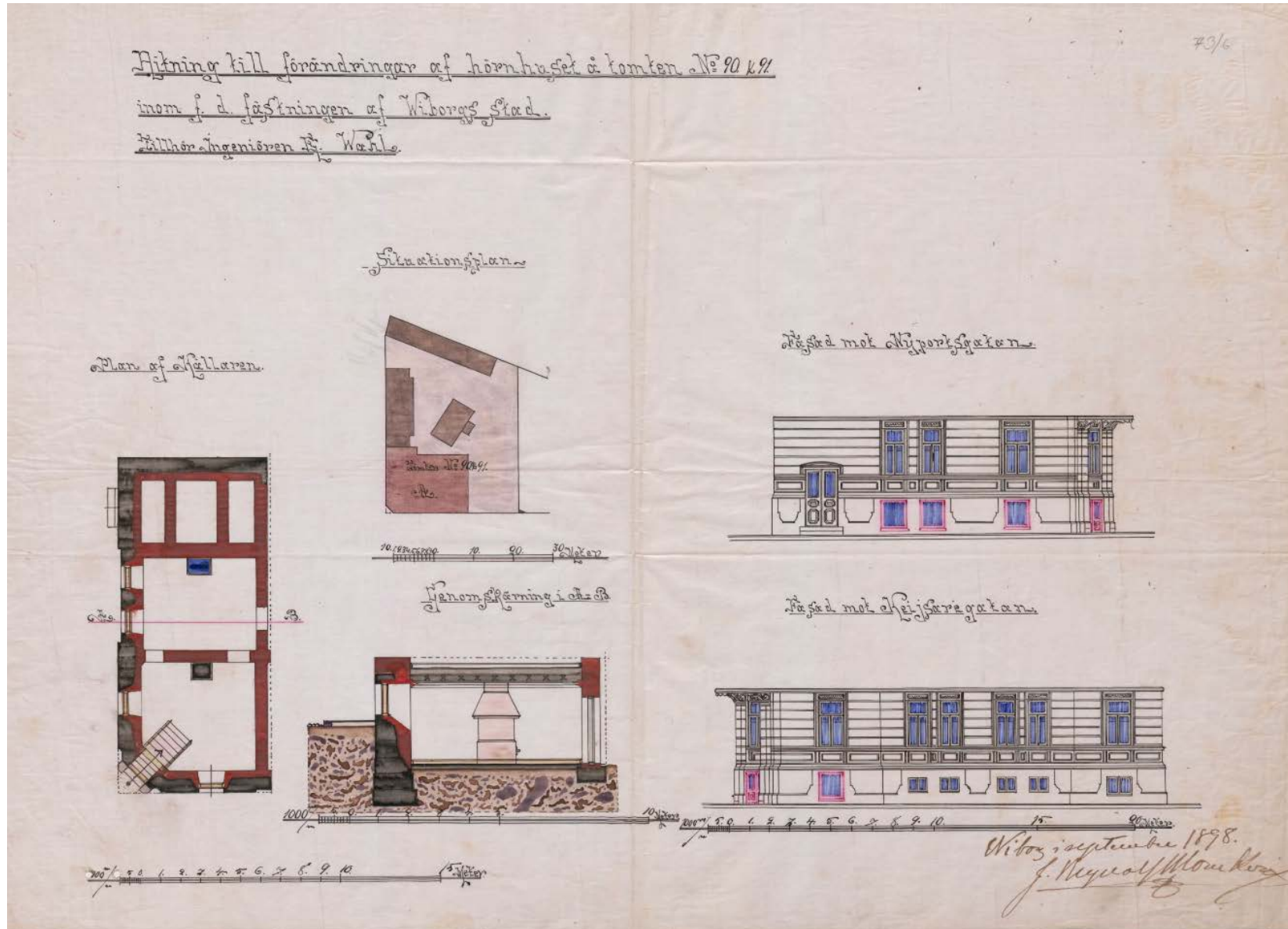
Илл. 8. Чертеж хозяйственного дома. Владение наследников Шабарина. 1898 г. // по Акту ГИКЭ выявленного ОКН «Жилой дом», ООО «Союзстройреставрация», 2016 г.
