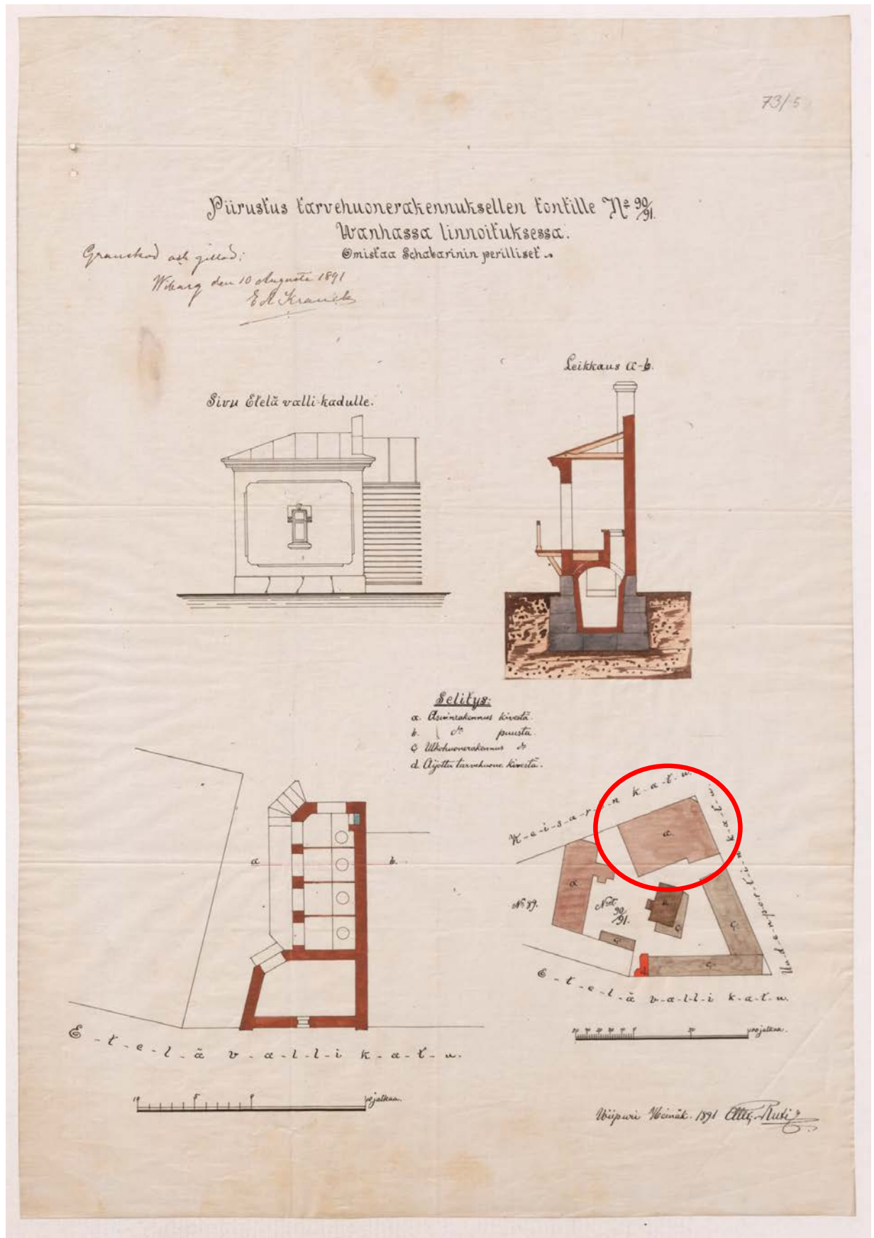
Илл. 7. Чертеж хозяйственного дома. Владение наследников Шабарина. 1891 г. // http://wiki.narc.fi/portti/images/4/45/Viipurinrakennuspiirustukset
