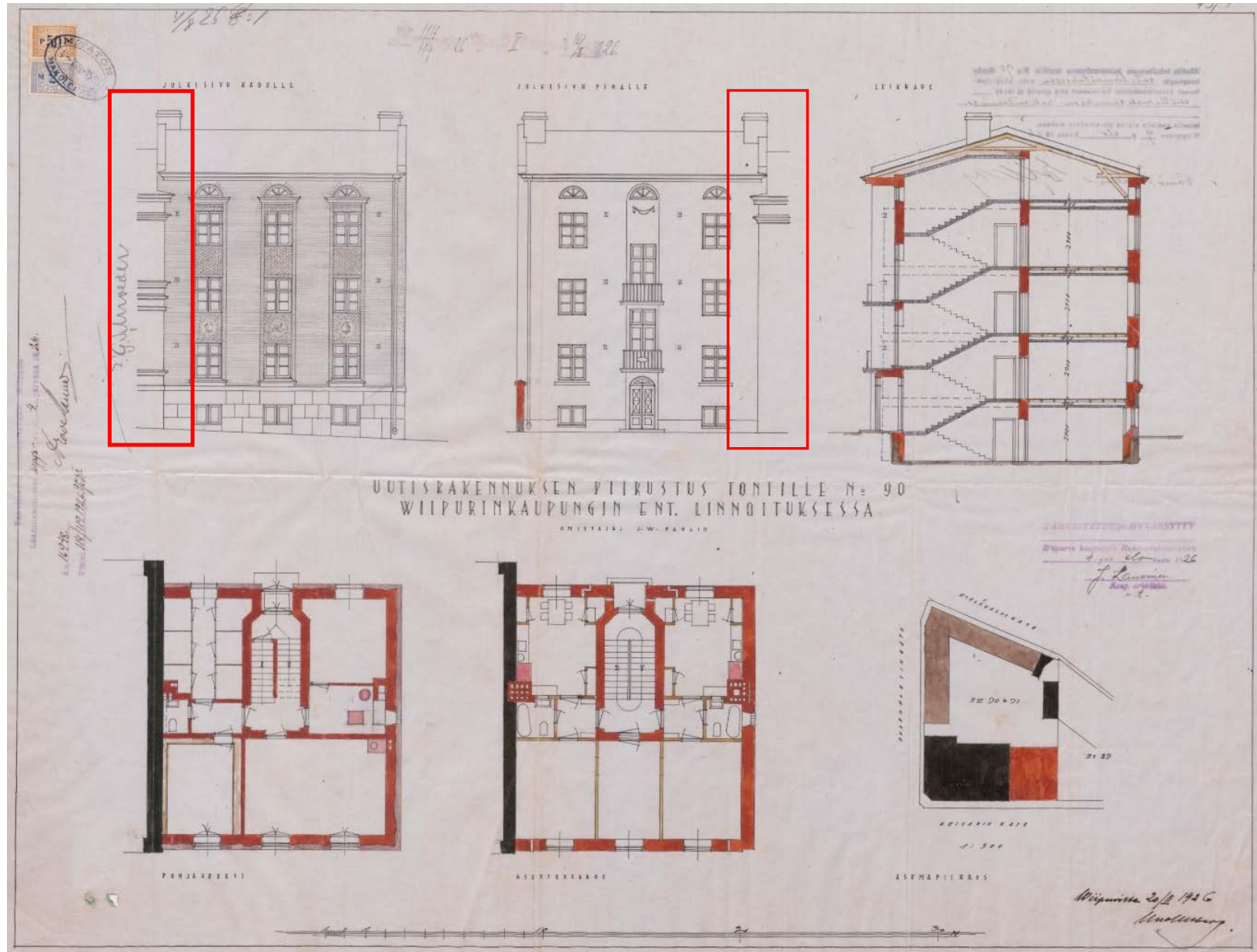
Илл. 9. Чертеж нового здания. Владение капитана Дж. В. Паулина. Архитектор Уно Ульберг..1926 г. // http://wiki.narc.fi/portti/images/4/45/Viipurinrakennuspiirustukset
