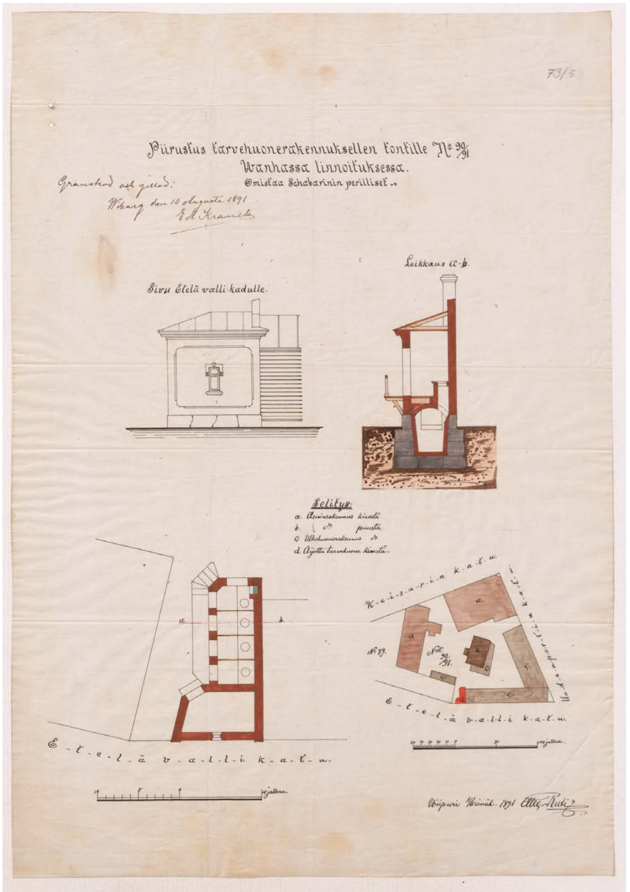
Илл. 9. Чертеж хозяйственного дома. Владение наследников Шабарина. 1891 г. // http://wiki.narc.fi/portti/images/4/45/Viipurinrakennuspiirustukset
