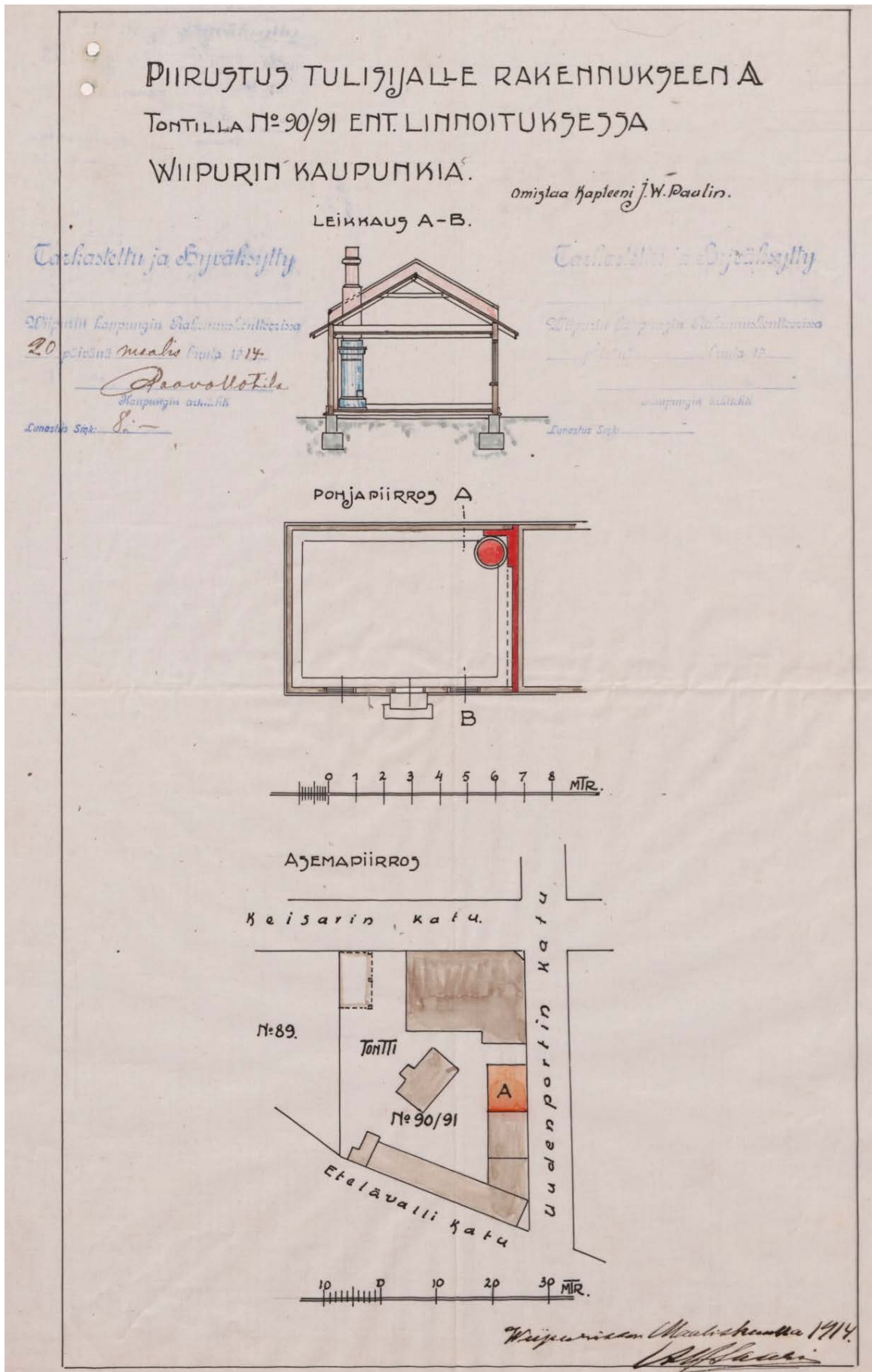
Илл. 11. Чертеж и планировка камина. Владение капитана Дж. В. Паулина. 1914 г. // http://wiki.narc.fi/portti/images/4/45/Viipurinrakennuspiirustukset
