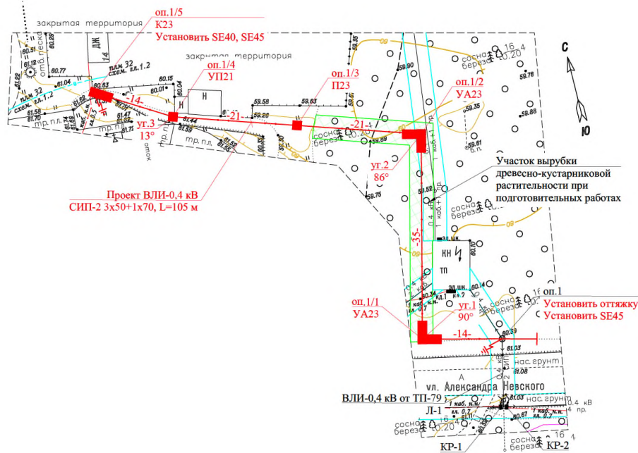
Илл. 13. Места установки опор согласно проектной документации
