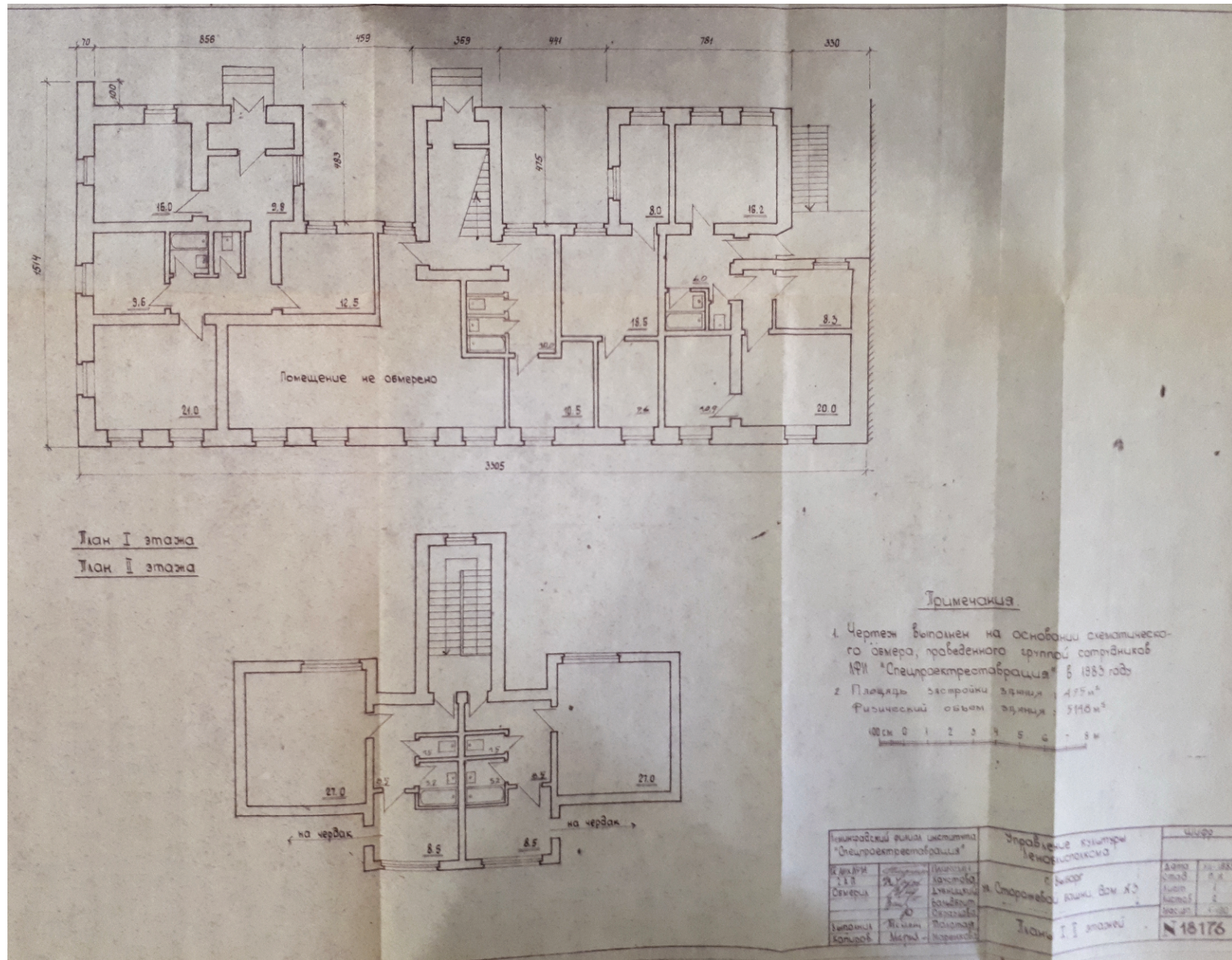
Илл. 11. План 1 и 2 этажей. Обмер. 1983 г. «г. Выборг. Жилой дом по ул. Старожевой башни, дом 3. Предварительные работы. Схематический обмер. Фотофиксация. Р. I, д. 1. НИ и ПИ «Спецпроектреставрация»//Архив ККЛО. № 1127-1
