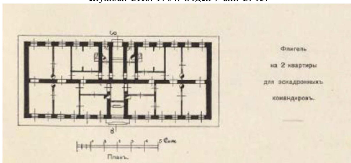
10. Нормальные планы казарменных построек в России. Дом для квартир эскадронных командиров. Воспроизводится по изданию: Барановский Г.В. Архитектурная энциклопедия второй половины XIX века Т. IV. Жилища службы. СПб. 1904. Отдел 9-ый. С. 15.
