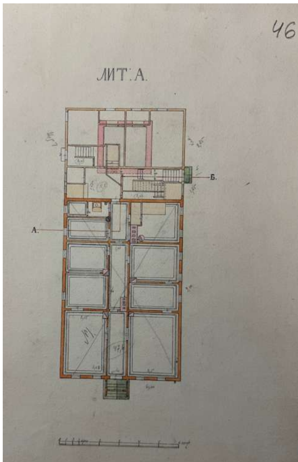
22. План первого этажа. 1889 г. ЦГИА СПб. Фонд 1546. Опись 5. Дело 32. Люцевская ул., N 62, Арсеньев В.В., (ранее Кузнецов А.Д., Кокорев)
