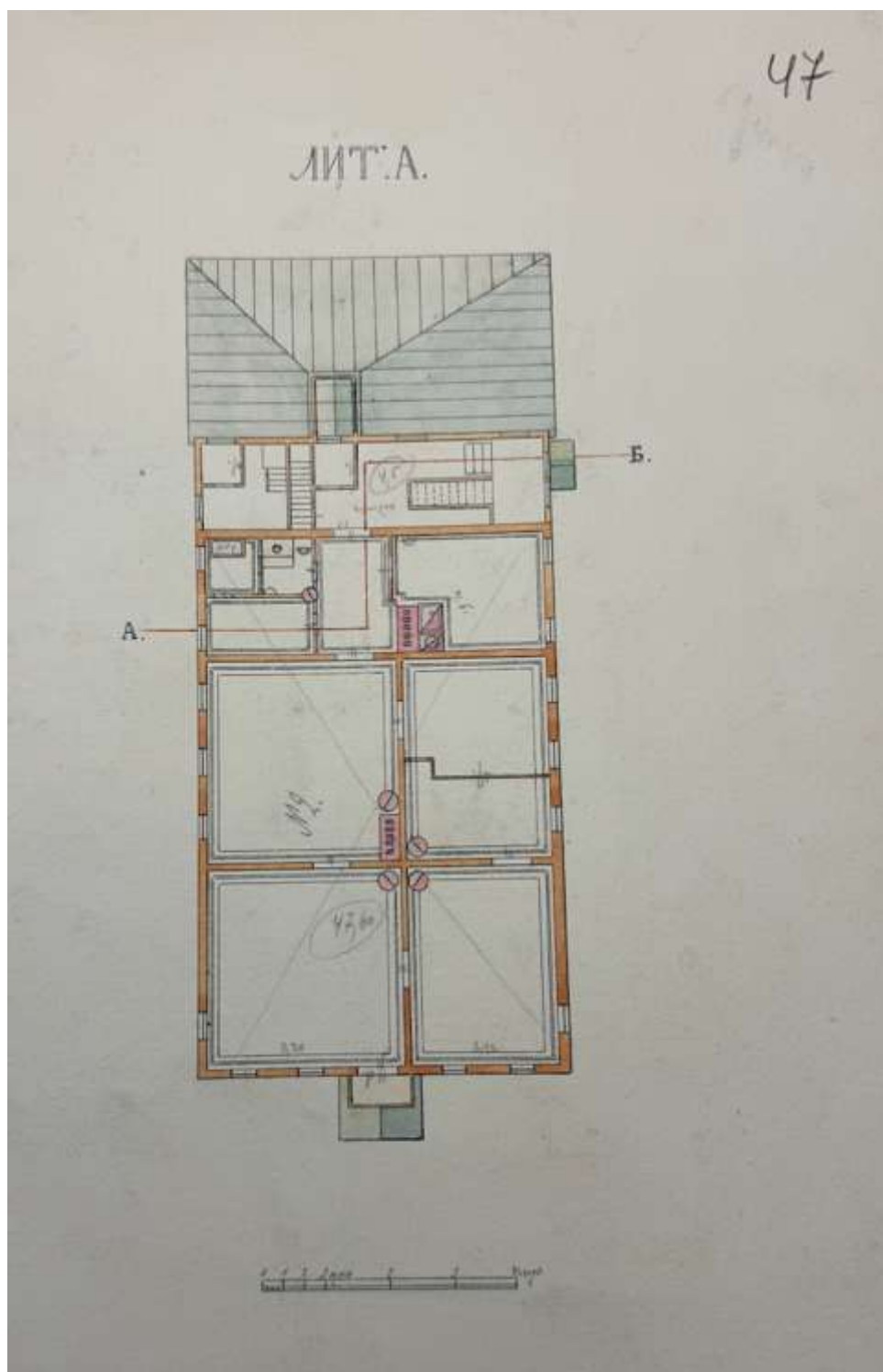
23. План второго этажа. 1889 г. ЦГИА СПб. Фонд 1546. Опись 5. Дело 32. Люцевская ул., N 62, Арсеньев В.В., (ранее Кузнецов А.Д., Кокорев)
