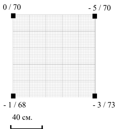
Рисунок 49.3. План шурфа № 3.
