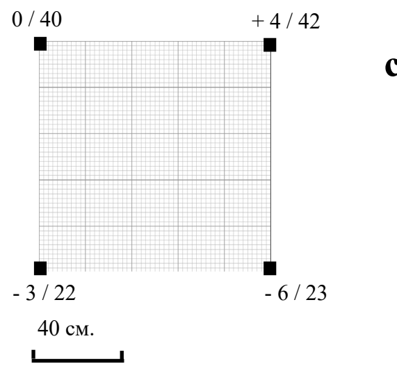
Рисунок 49.4. План шурфа № 4.
