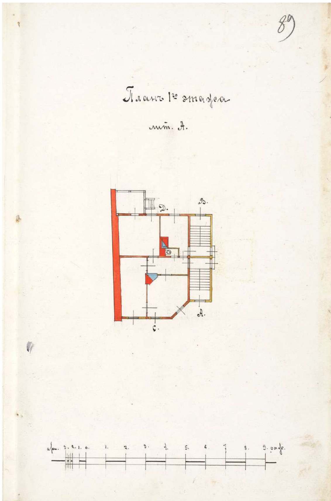
14. План 1-го этажа флигеля, обозначенного на плане двора под литерой А. РГИА. Фонд 491. Описание 4. Дело 1321
