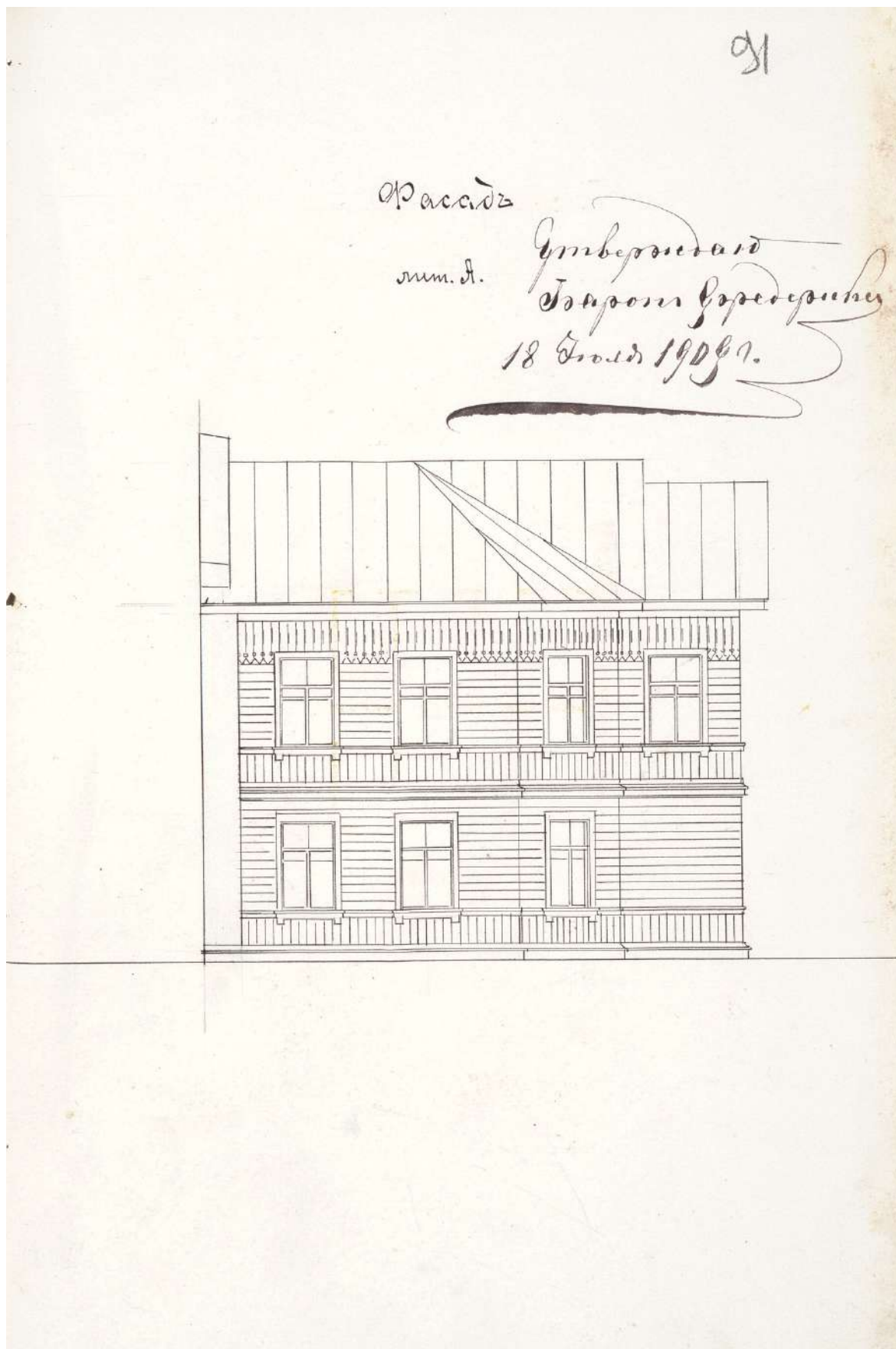
16. Фасад флигеля, обозначенного на плане двора под литерой А. РГИА. Фонд 491. Опись 4. Дело 1321
