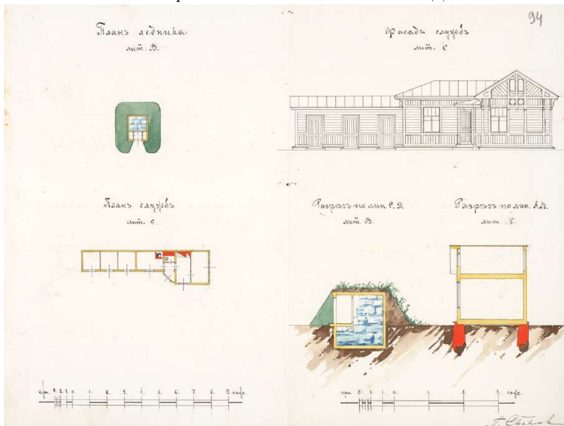
18. План ледника, план и фасад служб, разрезы. РГИА. Фонд 491. Опись 4. Дело 1321
