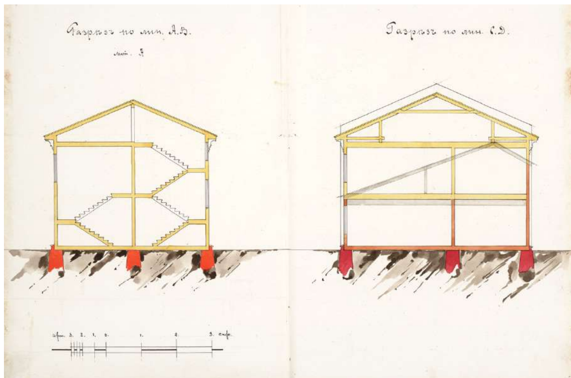
17. Разрезы флигеля по линиям АВ и СД, обозначенного на плане двора под литерой А. РГИА. Фонд 491. Опись 4. Дело 1321
