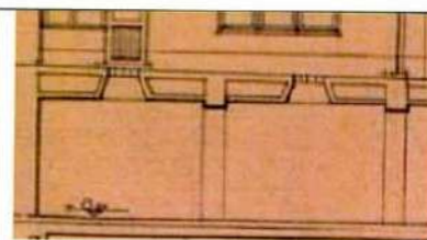
Конструкции световых фонарей в покрытии двора. Проект 1943 г.
