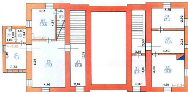
1 этаж
