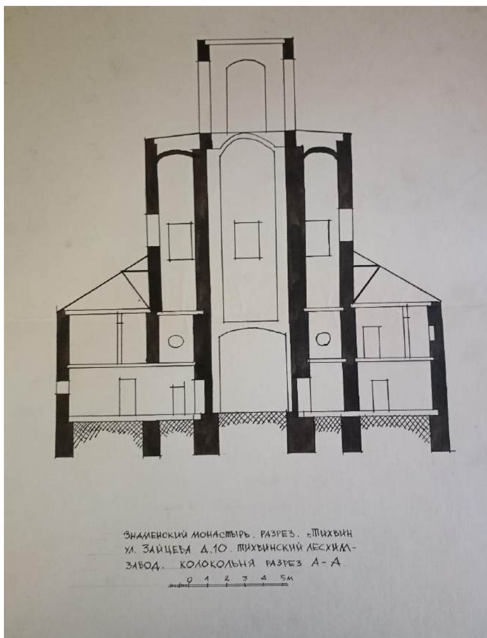
24. Тихвин. Введенский монастырь. Колокольня. Разрез. Состояние на конец XX в. АРХИВ КОМИТЕТА ПО СОХРАНЕНИЮ КУЛЬТУРНОГО НАСЛЕДИЯ ЛЕНИНГРАДСКОЙ ОБЛАСТИ. Инв. № 331.
