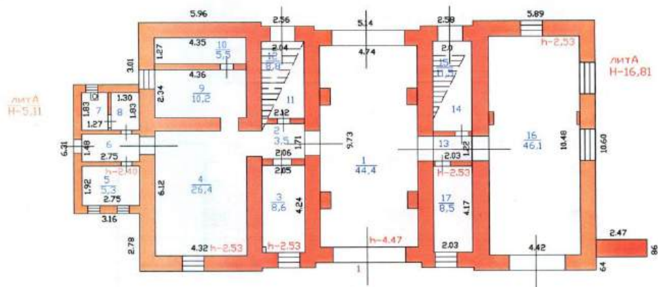
1 этаж
