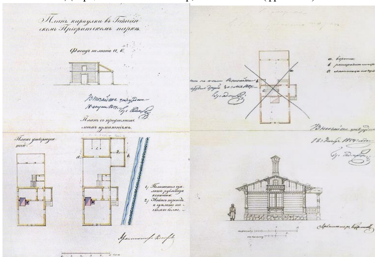
25. Кузьмин Р.И. Проект караулки в Приоратском парке. Фасады, план. 1854 г. Опубликовано: Петрова О.В. Архитектурная графика XIX в. Архив СПб ГБУК «ГМЗ «Гатчина». Инв. №№ ГДМ-263-ХІІ; ГДМ-276-ХІІ.
