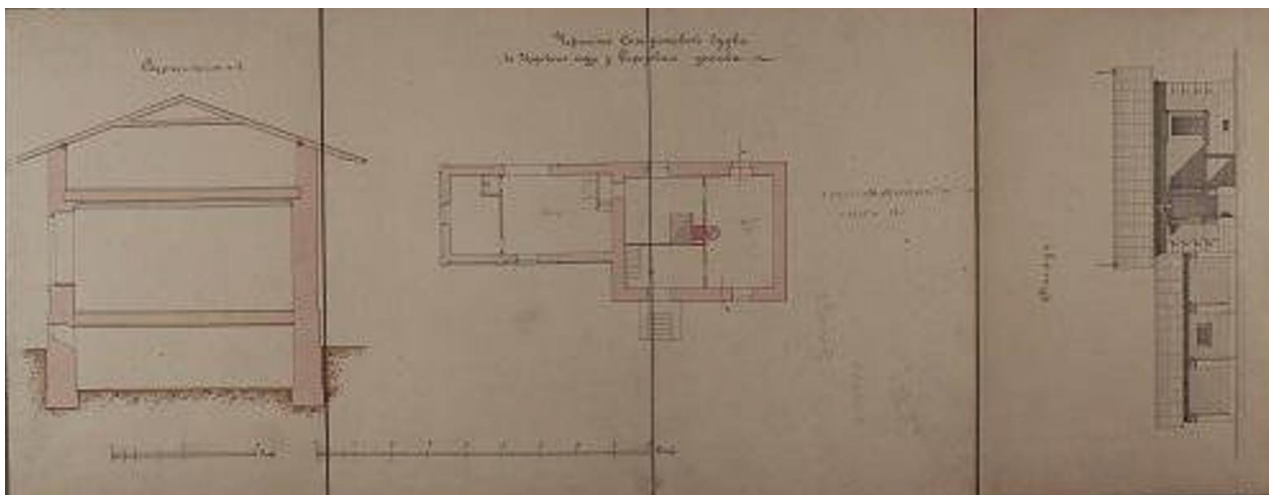
34. Разрез, план и фасад Сторожевой будки у Березового домика, из комплекта чертежей «Къ отчету за 1891 год». 1891 г. Санкт-Петербургское государственное бюджетное учреждение культуры "Государственный историко-художественный дворцово-парковый музей-заповедник "Гатчина". Инв. № ГДМ-68-ХII. Номер в государственном каталоге – 14024851.
