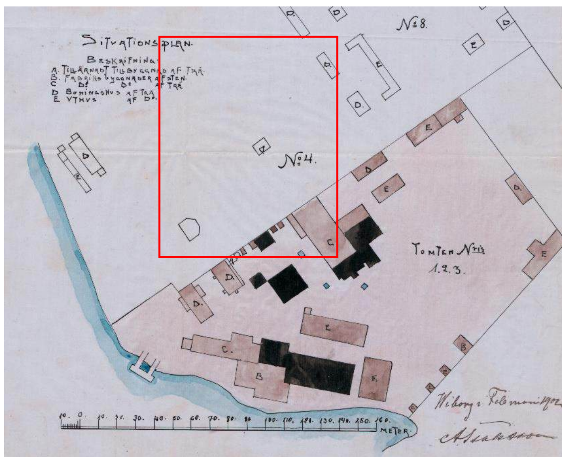
Илл. 5. Фрагмент ситуационного плана заводского участка. 1902 г.
