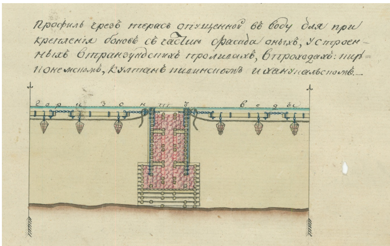
Конструкция бон, установленных в проливе между островами Суонионсари и Култанквисари. 1808 г. Источник: Национальный архив Финляндии.
