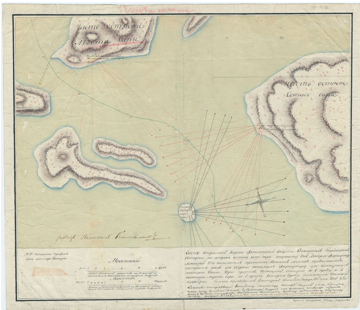
1808. Проект строительства двух батарей при редуте Култанкивисари, за подписью полковника Белокопытова. «Часть генеральной карты финляндской губернии с показанием возобновлённой батареи на острове Култан киви-сари ... и с наложением проекта какие ... предполагается построить вновь для обороны батареи на острове Сонин-Сари ... на 6 орудий и на острове Муста-сари на 5 орудий, которые орудия доставить из Выборга. Сочинена при выборгской инженерной команде генваря 25 дня 1808 г. Инженер полковник Белокопытов». Источник: Финский национальный архив digi.narc.fi
