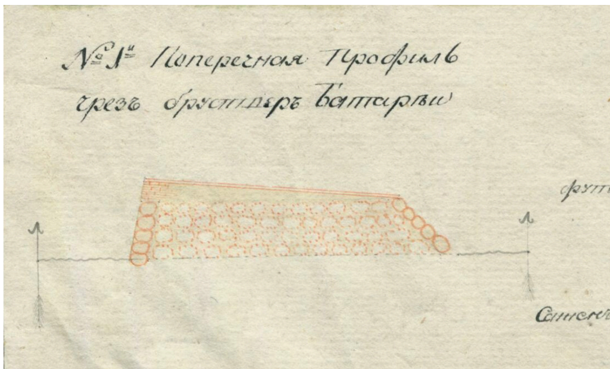
Поперечный разрез бруствера батареи на острове Суонионсаари. Проект. 1808 г. Фрагмент Генеральной карты финляндской губернии. Источник: Национальный архив Финляндии.
