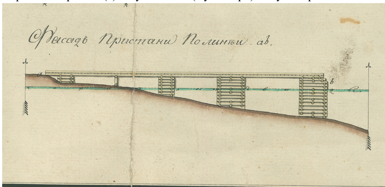
Причал, построенный к батарее Суонионсаари. 1808 г. Источник: Национальный архив Финляндии.
