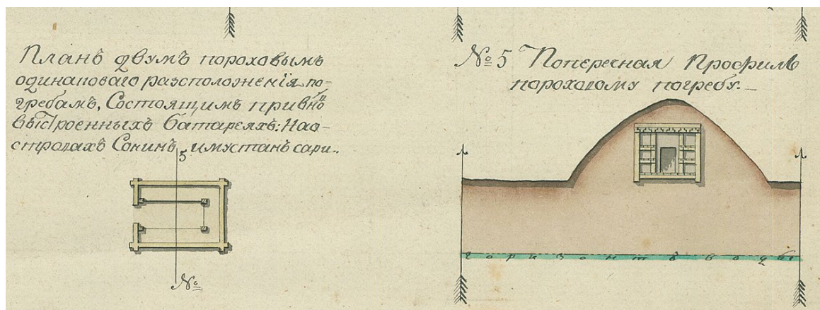
Пороховой снарядный погреб при батарее Суонионсари. Фрагмент генплана. 1808 г. Источник: Национальный архив Финляндии.
