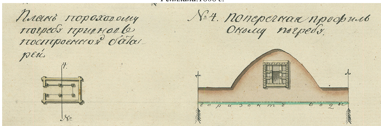
Конструкция порохового погреба батареи. 1808 г.
