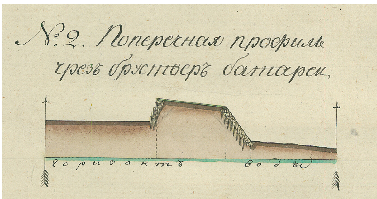
Конструкция земляного вала батареи Кирккониеми. Фрагмент Генплана укреплений. 1808 г. Источник: цифровой фонд Национального архива Финляндии.
