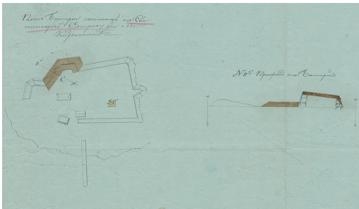
Ремонт редута Киркониemi, разрушенного штормом. Генплан с показанием «перестроенного вновь» порохового погреба и поперечный разрез бруствера. 1811 г. Источник: цифровой фонд Национального архива Финляндии.
