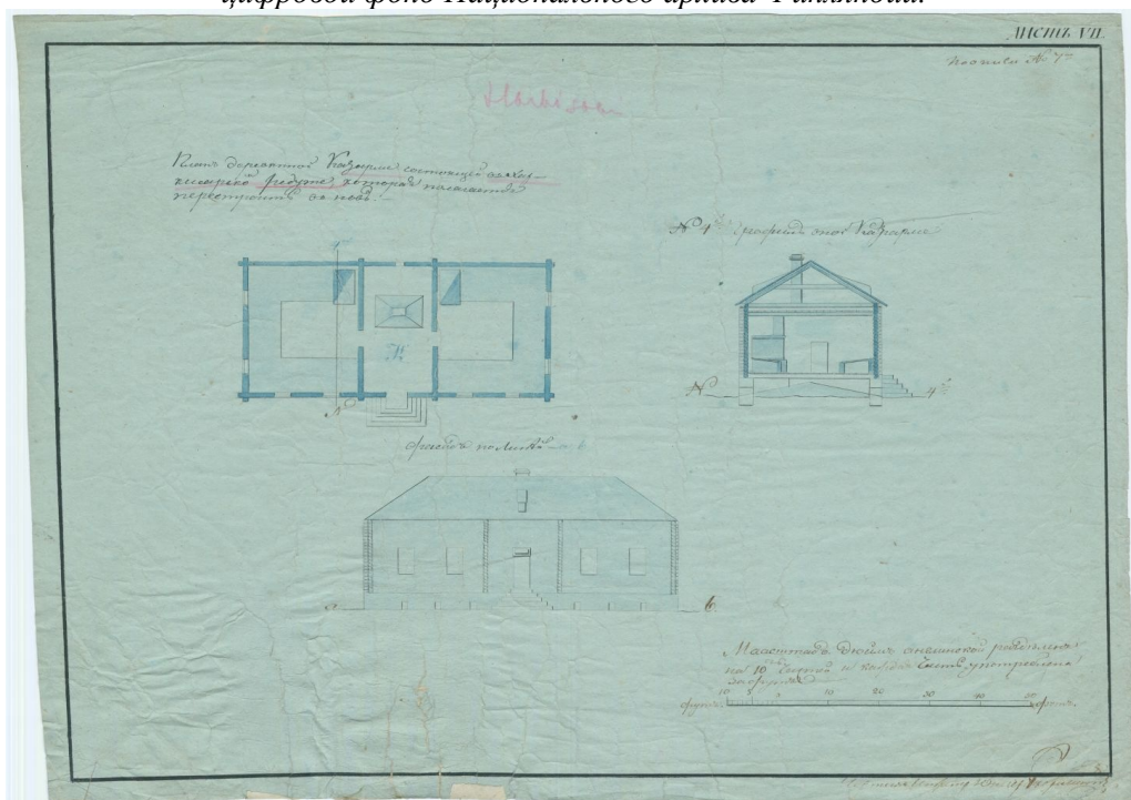
План деревянной казармы состоящей харкисарского редута, которая предполагается построить заново. 1821 год. Источник: цифровой фонд Национального архива Финляндии.
