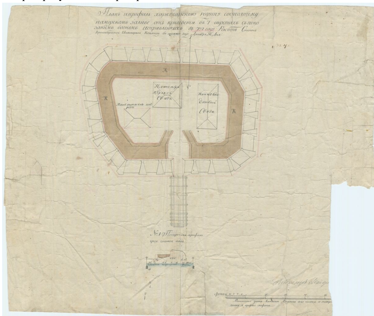
План профиль харкисарского редута состоящему на морском заливе от крепости в 7 верстах (...) 1797 г. Источник: цифровой фонд Национального архива Финляндии.
