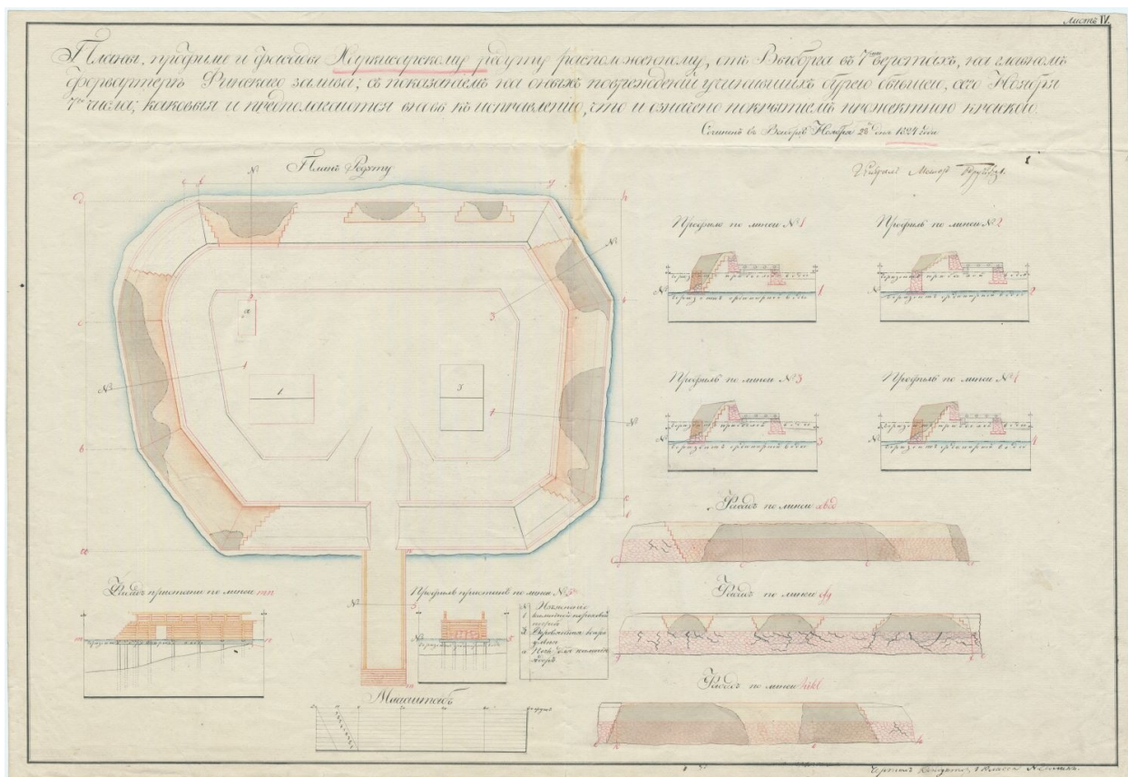
Планы, профили и фасады Харкисарскому редуту, расположенному от Выборга в 7 верстах на главном фарватере Финского залива, с показанием повреждений, учиненных бурей ноября 7 числа 1824 года. Источник: цифровой фонд Национального архива Финляндии.
