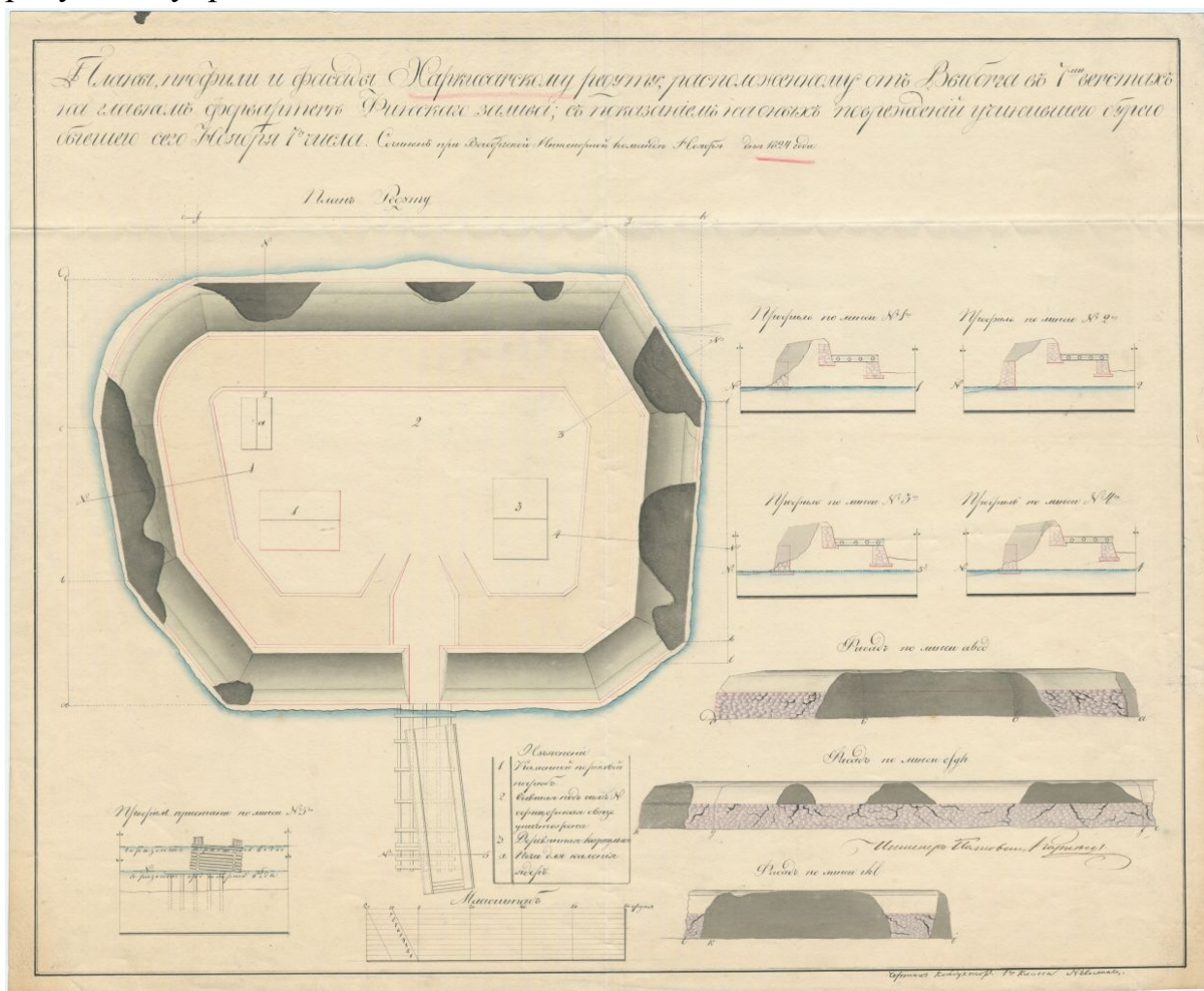
Планы, профили и фасады Харкисарскому редуту, расположенному от Выборга в 7 верстах на главном фарватере Финского залива, с показанием повреждений, учиненных бурей ноября 7 числа 1824 года. Источник: цифровой фонд Национального архива Финляндии.
