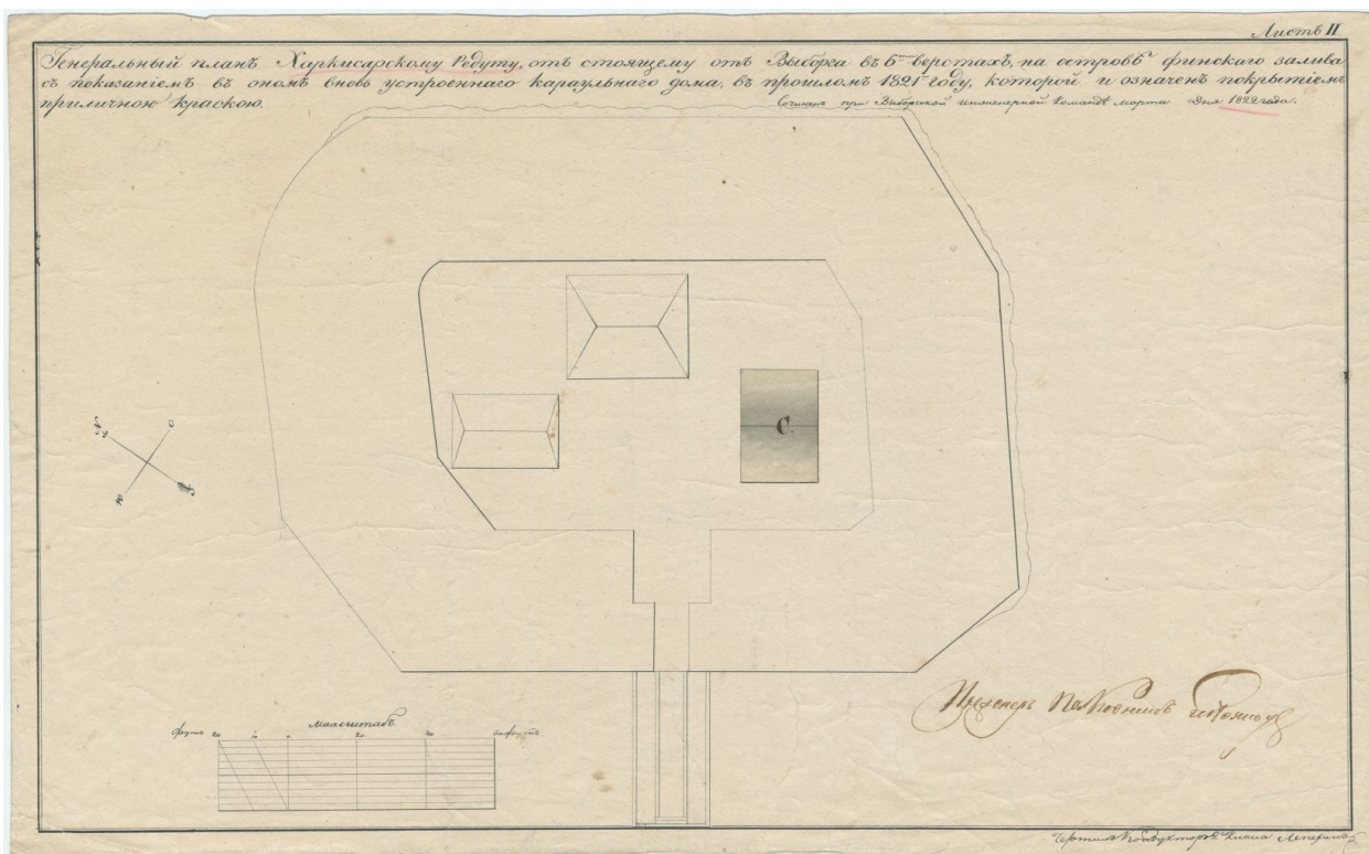
Генеральный план Харкисарскому редуту (...). Марта 1822 года. Источник: цифровой фонд Национального архива Финляндии.
