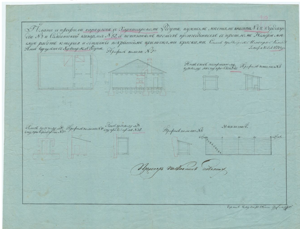
Планы и профили караульни в Харкисарском редуте (...), 10 декабря 1821 года. Источник: цифровой фонд Национального архива Финляндии.
