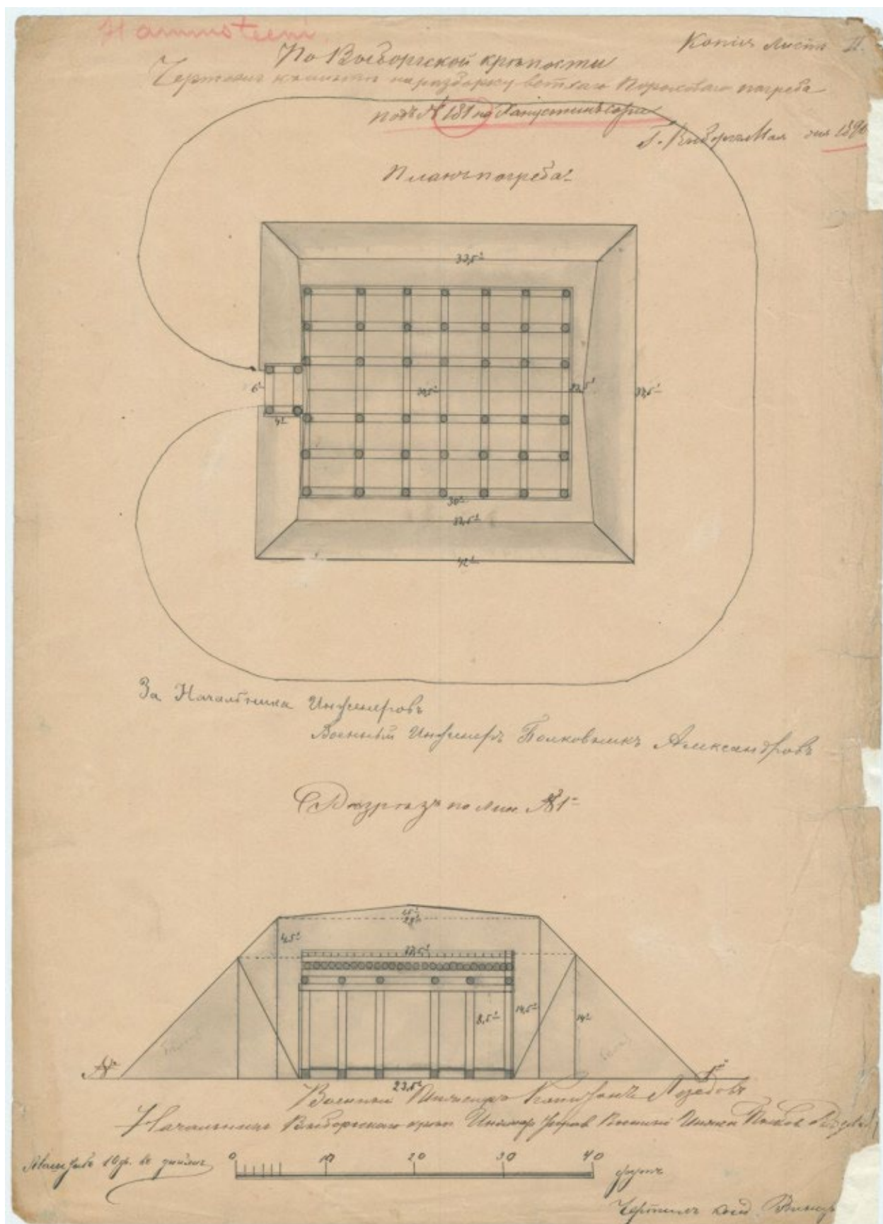
Чертеж порохового погреба под №181 на Ханнустиенсаари. г. Выборг, 1890 г. Источник: Цифровой фонд Национального архива Финляндии.
