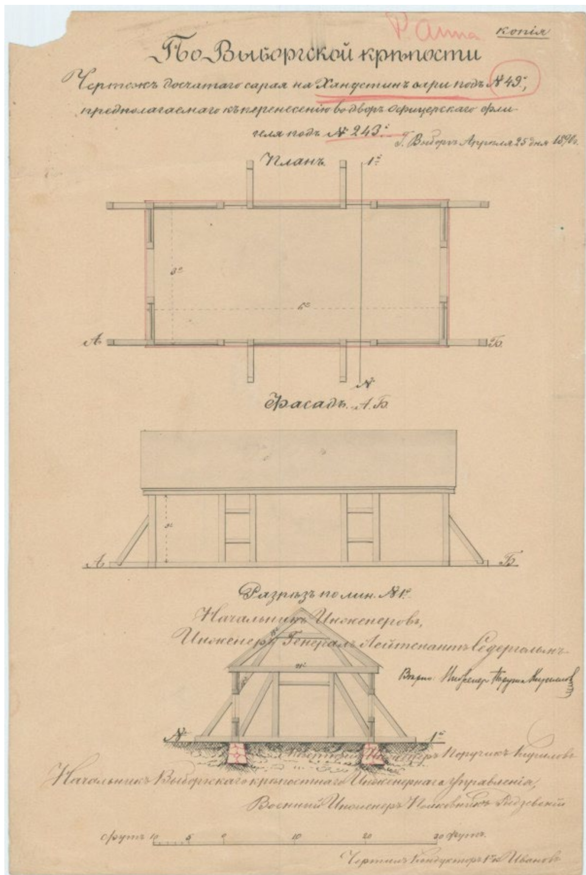
Чертеж дощатого сарая №185 на Хангустиненсаари под №49 предлагаемого к перенесению во двор офицерского флигеля №243. г. Выборг, 1891 г. Источник: Цифровой фонд Национального архива Финляндии.
