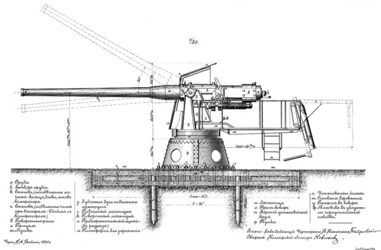
Общий вид установки Канэ. 1900 г.
