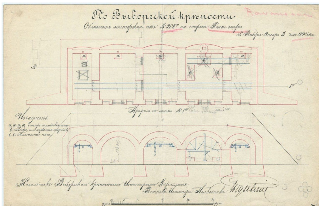
Чертеж обливочной мастерской на о. Равансаари. г. Выборг, 1890 г. Источник: Национальный архив Финляндии.
