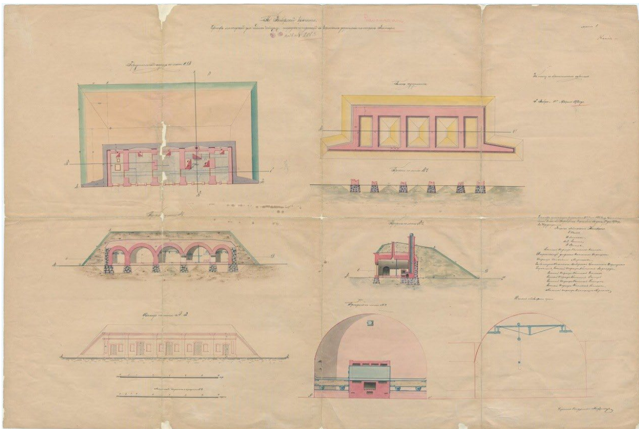
Чертеж каменной обливочной мастерской на о. Равансаари. 1883 г. Источник: Национальный архив Финляндии.
