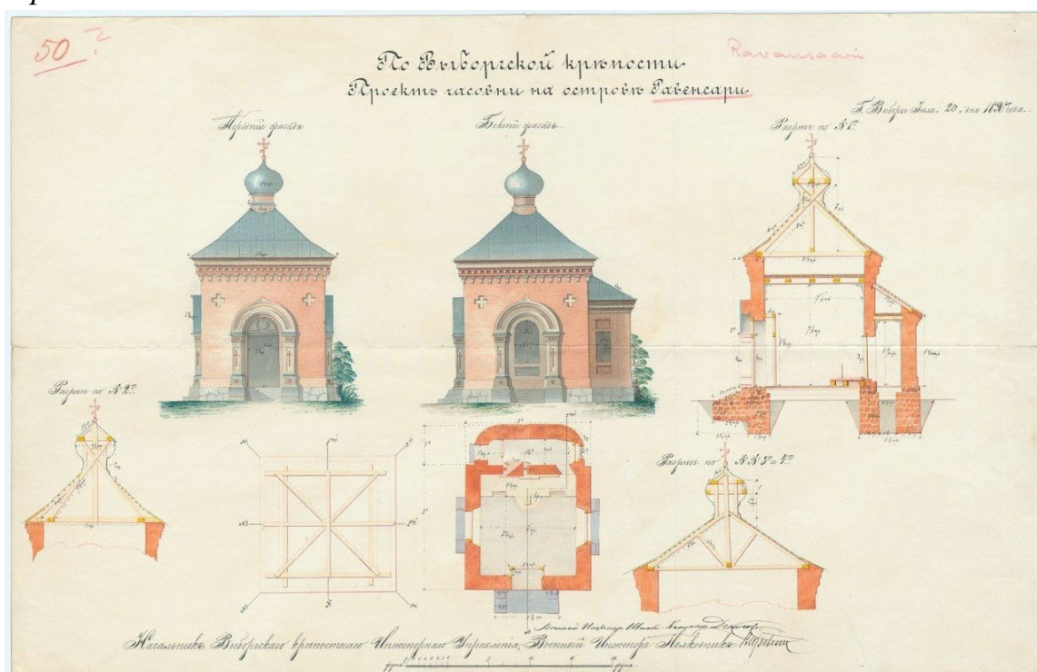
Проект часовни на острове Равансаари. г. Выборг, 1907 г. Источник: архив провинции Миккели (Mikkelin maakunnan arkisto, MMA), Финляндия 8/KS:6.
