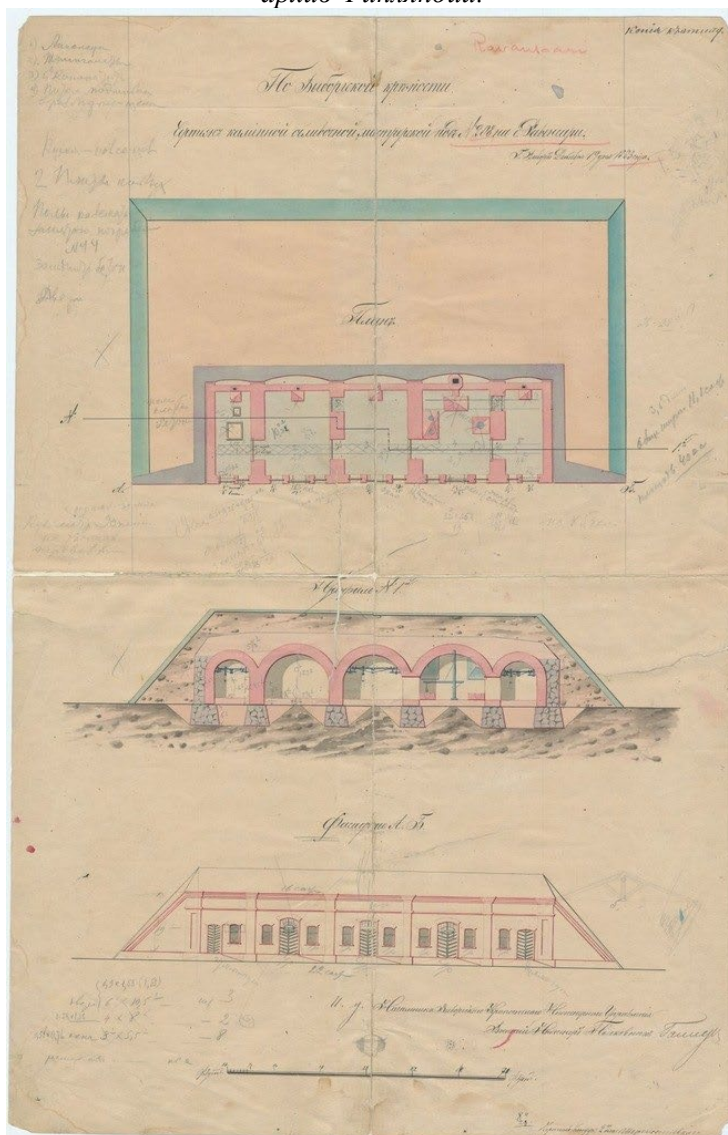
Чертеж каменной обливочной мастерской на о. Равансаари. 1883 г. Источник: Национальный архив Финляндии.
