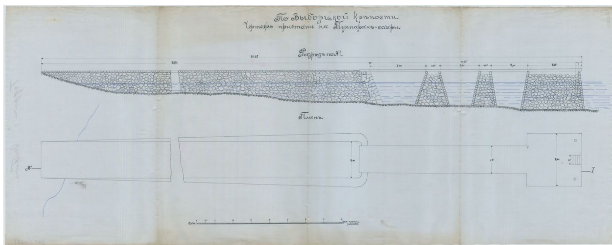
Чертеж пристани на Туппурансаари. Документ из цифровых фондов Национального архива Финляндии.
