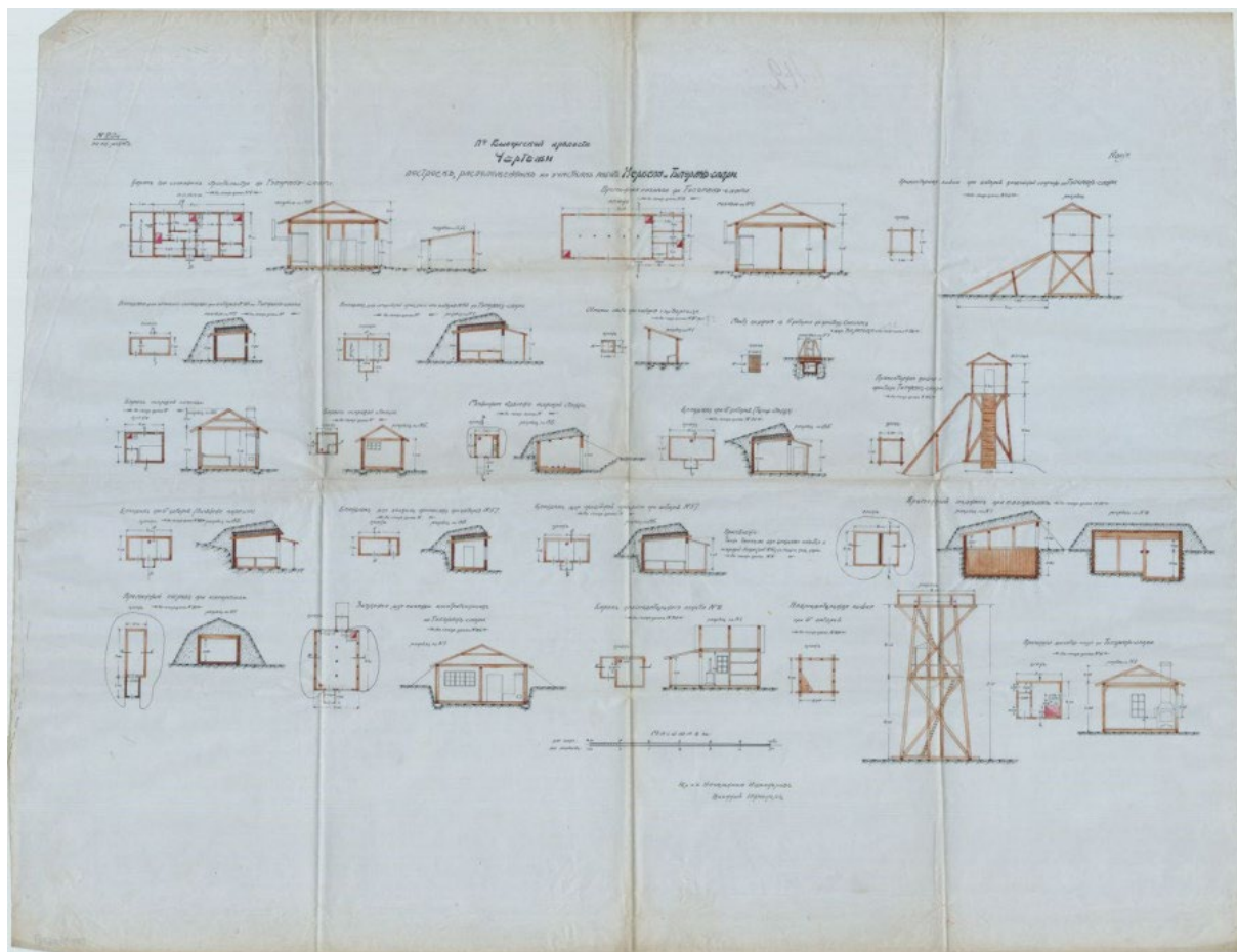
Чертеж построек, расположенных на о.Туппурансаари. Документ из цифровых фондов Национального архива Финляндии.
