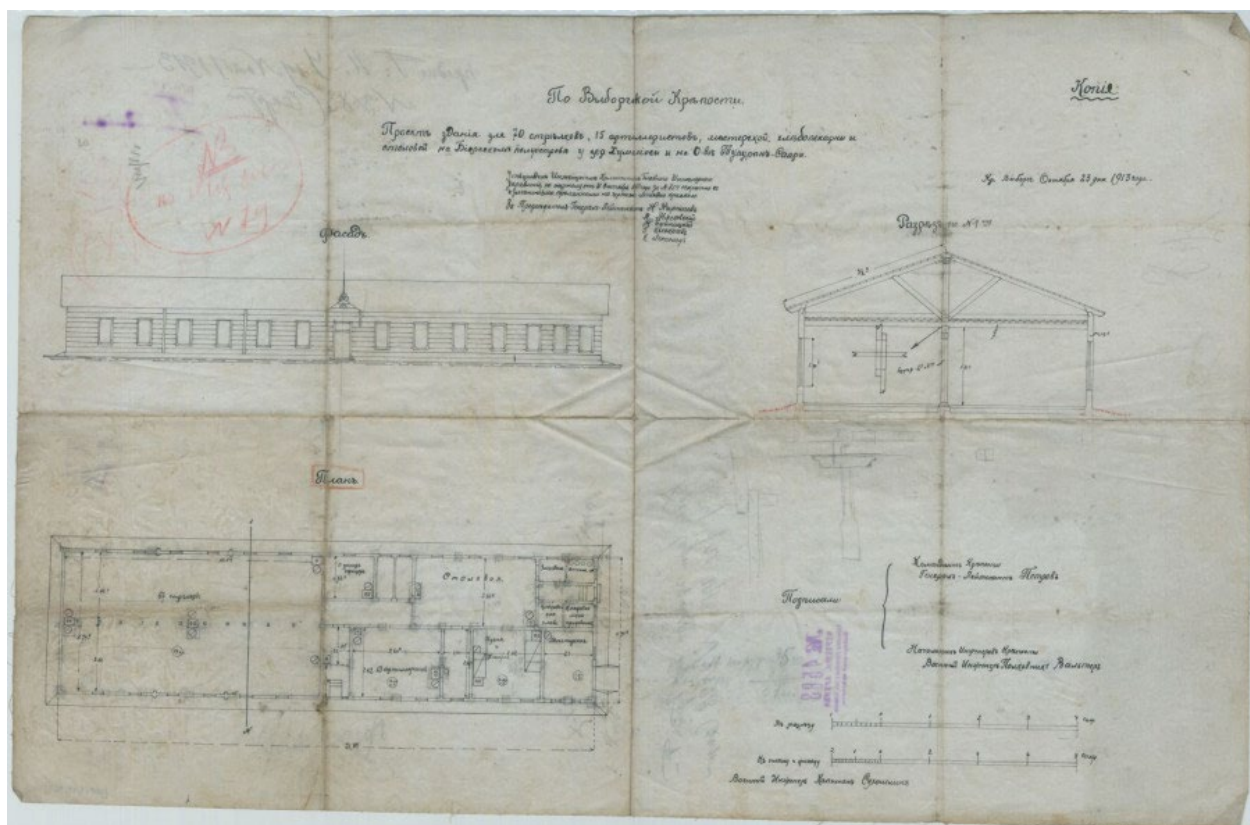
Проект здания для 70 зрителей, 15 артиллеристов, мастерской, кладовыми и столовой на острове Туппурансаари. г. Выборг, 1913 г. Документ из цифровых фондов Национального архива Финляндии.
