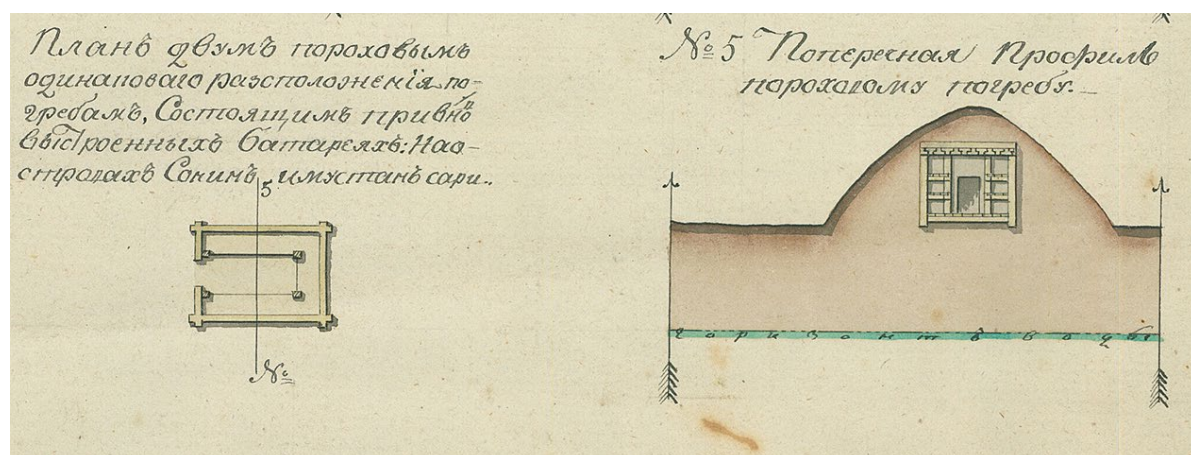
Конструкция порохового погреба на о. Муста-сари. 1808 г. Источник: Национальный архив Финляндии.
