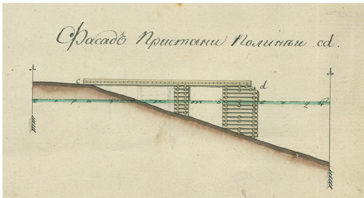
Деревянный причал у острова Муста-сари. 1808 г. Источник: Национальный архив Финляндии.
