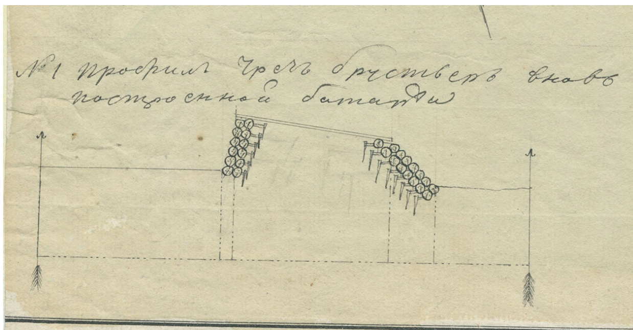
Конструкция бруствера построенной батареи на о.Муста-сари. Черновой вариант. 1808 г. Источник: Национальный архив Финляндии.
