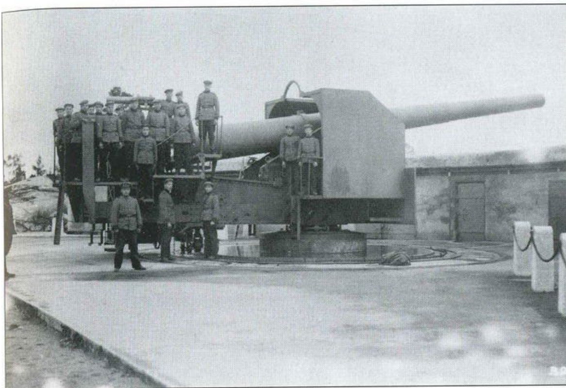
254-мм пушка на станке Дурляхера, переделанная финнами Пушка на станке Дурляхера калибра 254 мм. Источник: www.zwezet.turbina.ru
