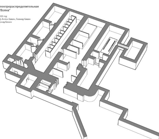
Подземная электроподстанция в Лемболово. 1933 г.
