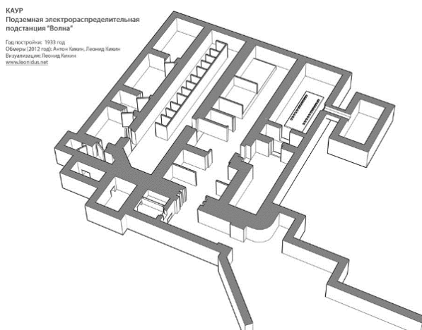
Подземная электростанция в Лемболово. 1933 г. Источник: https://www.aroundspb.ru
