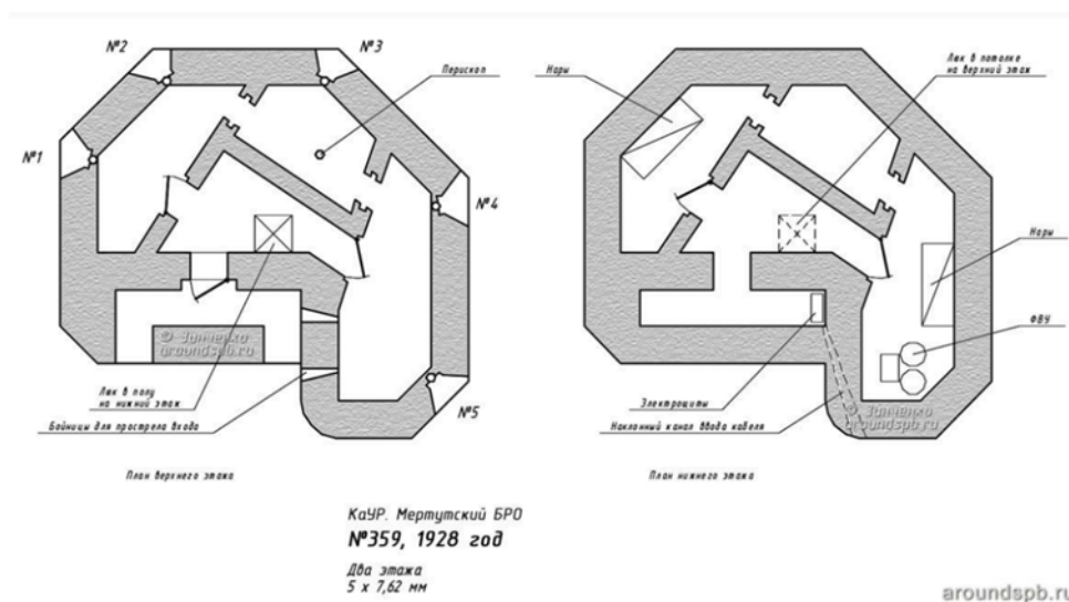
Поэтажный план ДОТа №359
