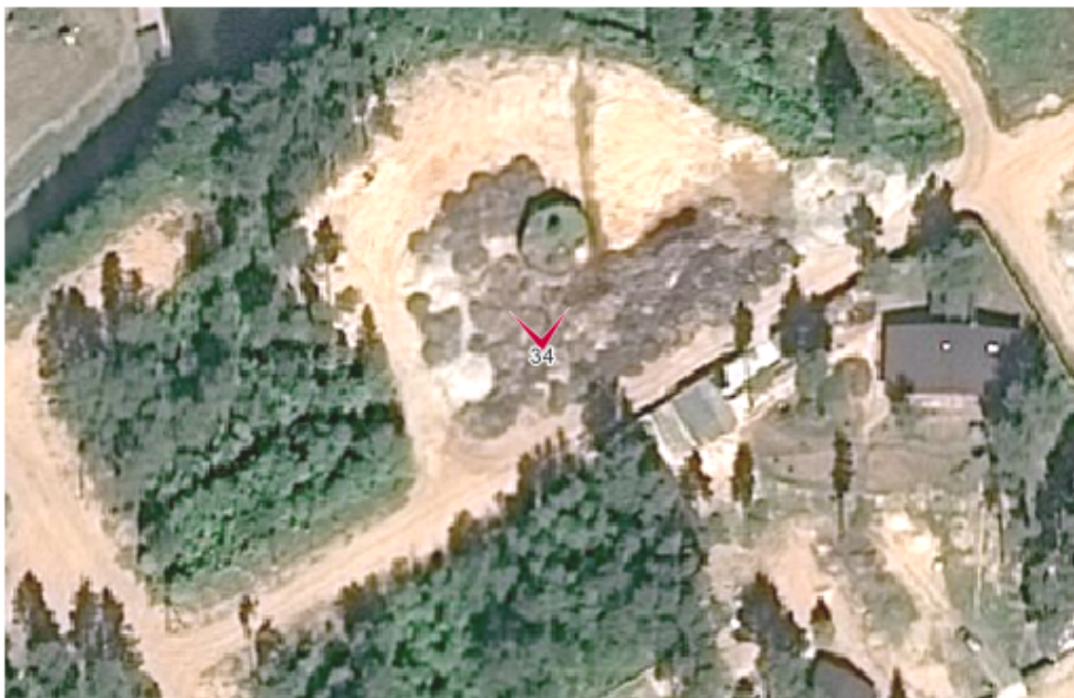
Фото 34. Выявленный объект культурного наследия « Карельский укрепленный район. Мертутьский батальонный район обороны. Пулеметная огневая точка ДОТ № 359». Направление съемки север.
