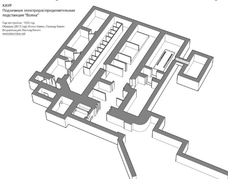
Подземная элетроподсатнция в Лемболово. 1933 г. Источник: https://www.aroundspb.ru
