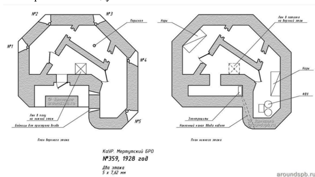
Поэтажный план ДОТа №359
