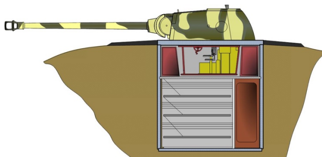
Строение танковой огневой точки
