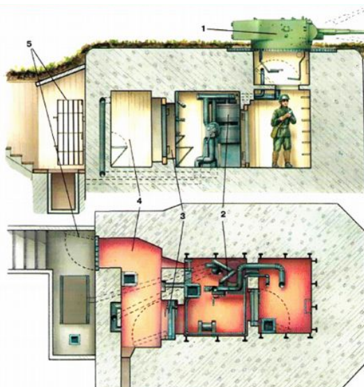
ДОТ с башней танка Т-26, 1940-е гг.
