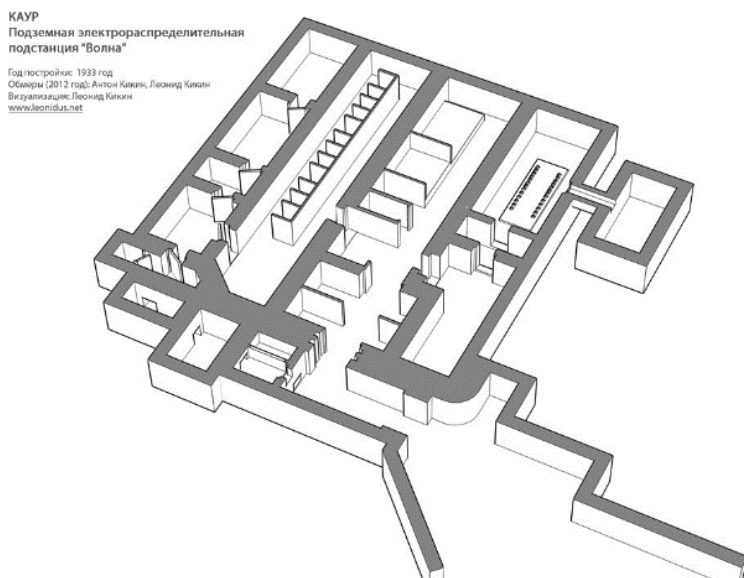
Подземная электроподстанция в Лемболово. 1933 г.
