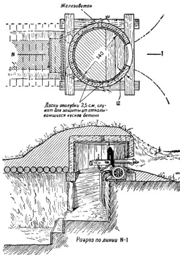
План и разрез ЖБОТа. Источник https://topwar.ru
