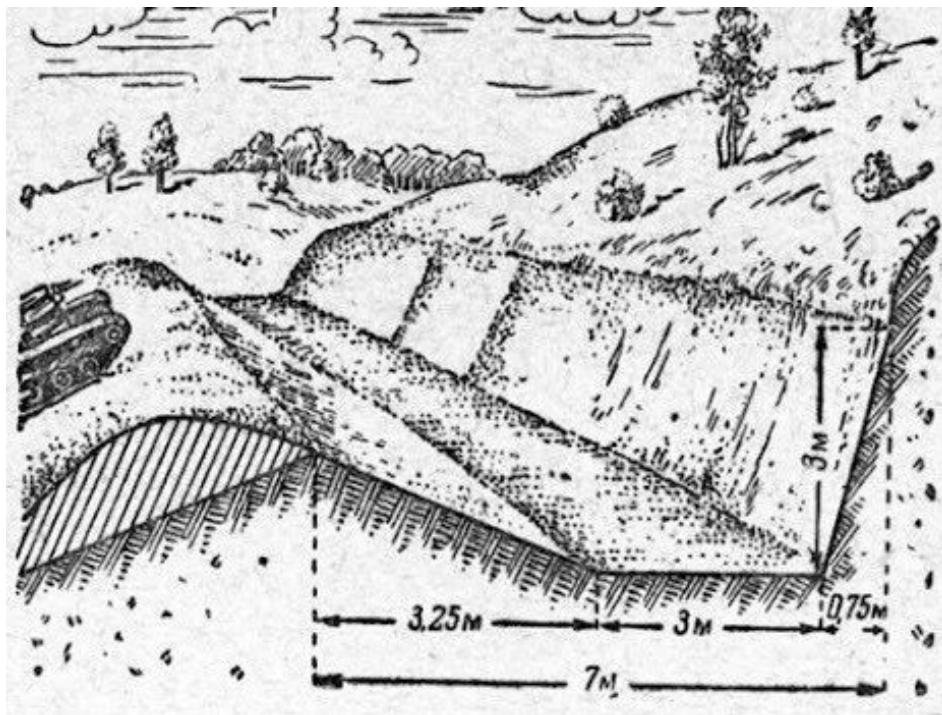
Противотанковый эскарп. Источник: https://dzen.ru
