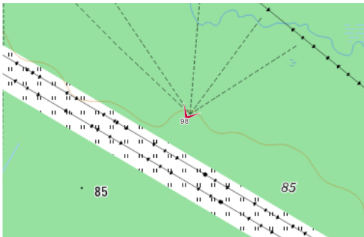
Фото 98. Выявленный объект культурного наследия « Карельский укрепленный район. Меднозаводский батальонный район обороны. Фортификационный комплекс (пулеметная огневая точка ДОТ № 333, № 337, № 341, ЖБОТ, эскарп, противотанковые надолбы)». Вид на ДОТ № 341. Направление съемки северо-восток.
