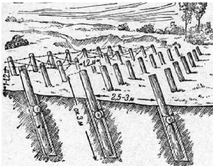
Примерная схема установки деревянных надолб. Источник: https://dzen.ru
