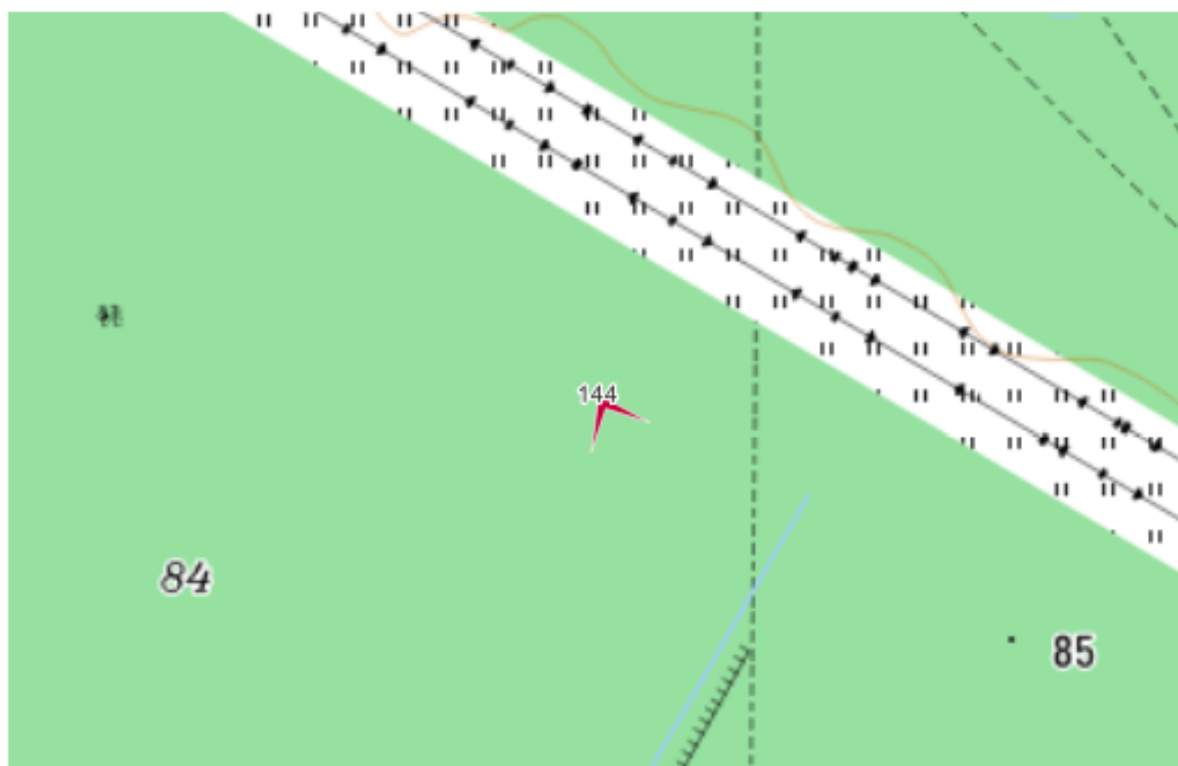
Фото 144. Выявленный объект культурного наследия « Карельский укрепленный район. Меднозаводский батальонный район обороны. Фортификационный комплекс (пулеметная огневая точка ДОТ № 333, № 337, № 341, ЖБОТ, эскарп, противотанковые надолбы)». Вид на надолбы. Направление съемки юго-восток.
