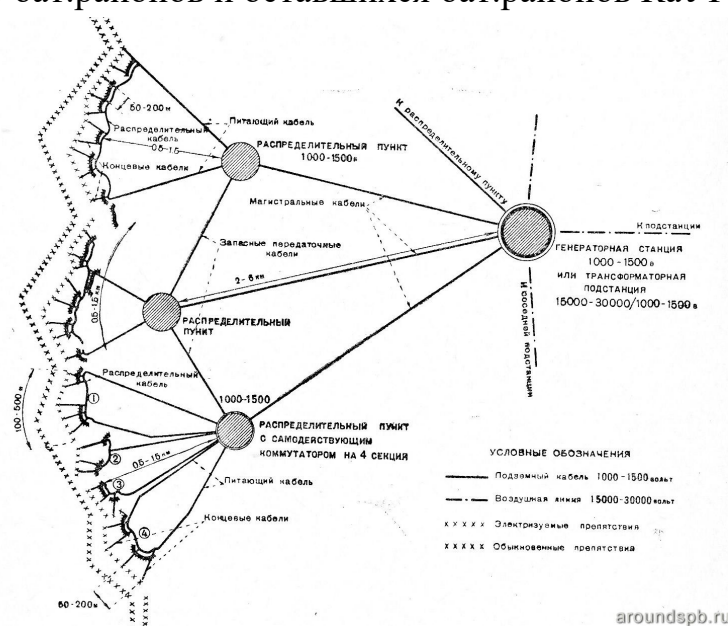
Схема сети питающих проводов (на примере Лемболовского батрайона). 1938 год. Источник: https://www.aroundspb.ru/
