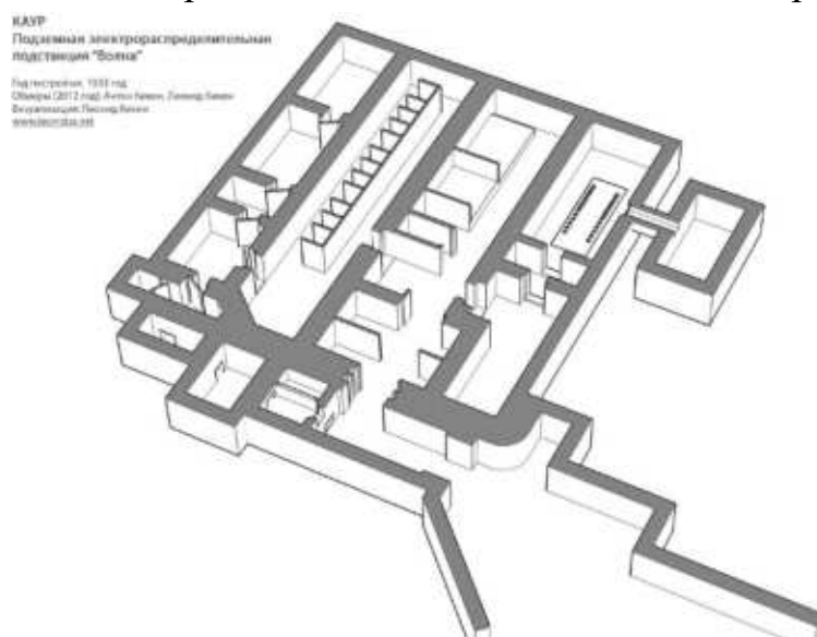
Подземная электроподстанция в Лемболово. 1933 г. Источник: https://www.aroundspb.ru
