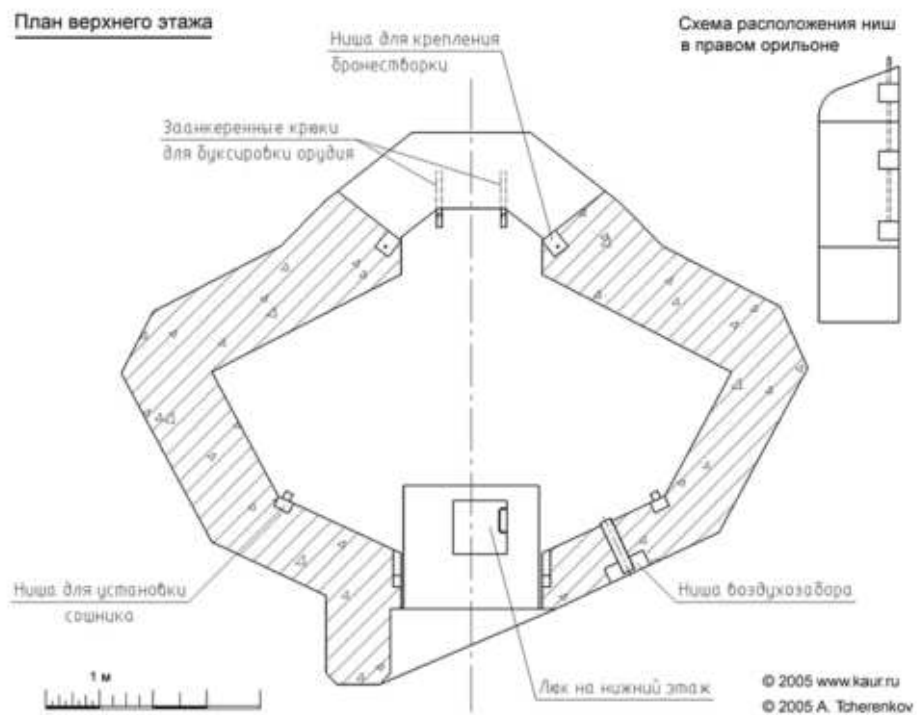
План верхнего этажа и разрез по линии Б-Б северо-восточного каземата батареи. Источник: https://www.kaur.ru
