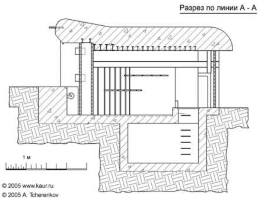
План верхнего этажа и разрез по линии А-А северо-восточного каземата батареи. Источник: https://www.kaur.ru
