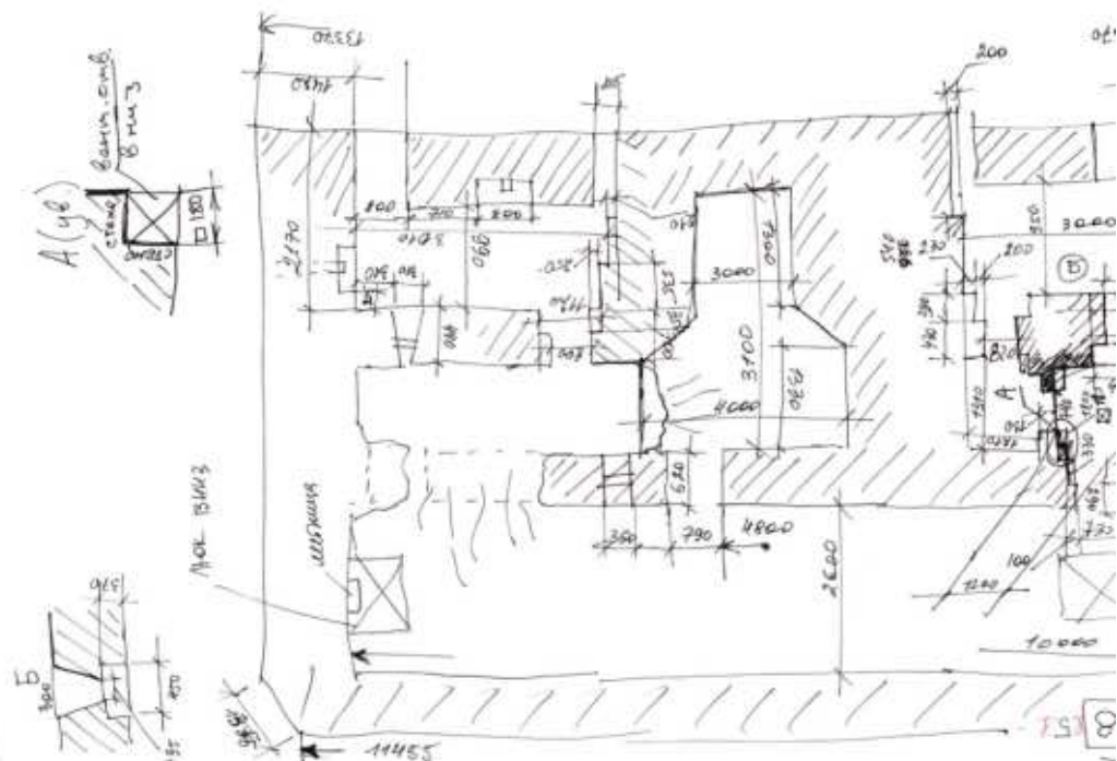
8 Верхний этаж. Казематированный этаж
