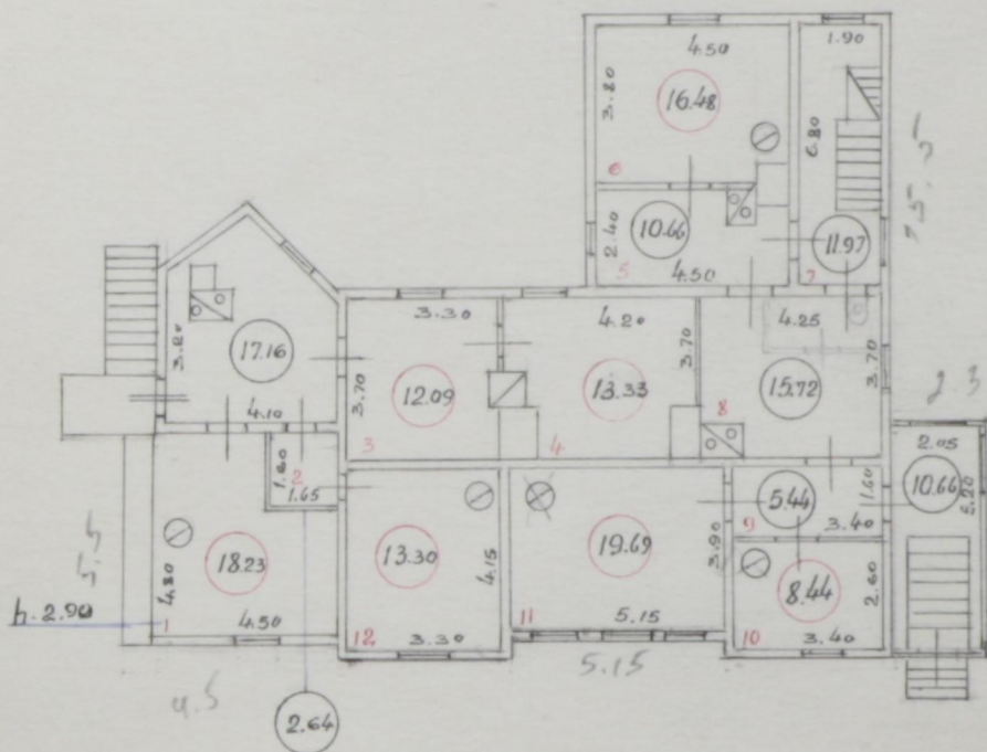
План 1 этажа
