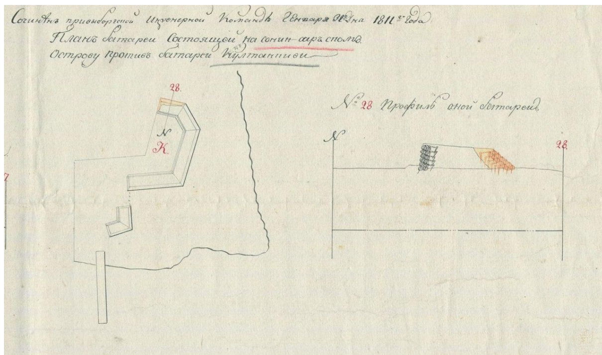
Разрушение редута Суонионсари в результате штурма и проект восстановления бруствера. 1811 г. Источник: Национальный архив Финляндии.
