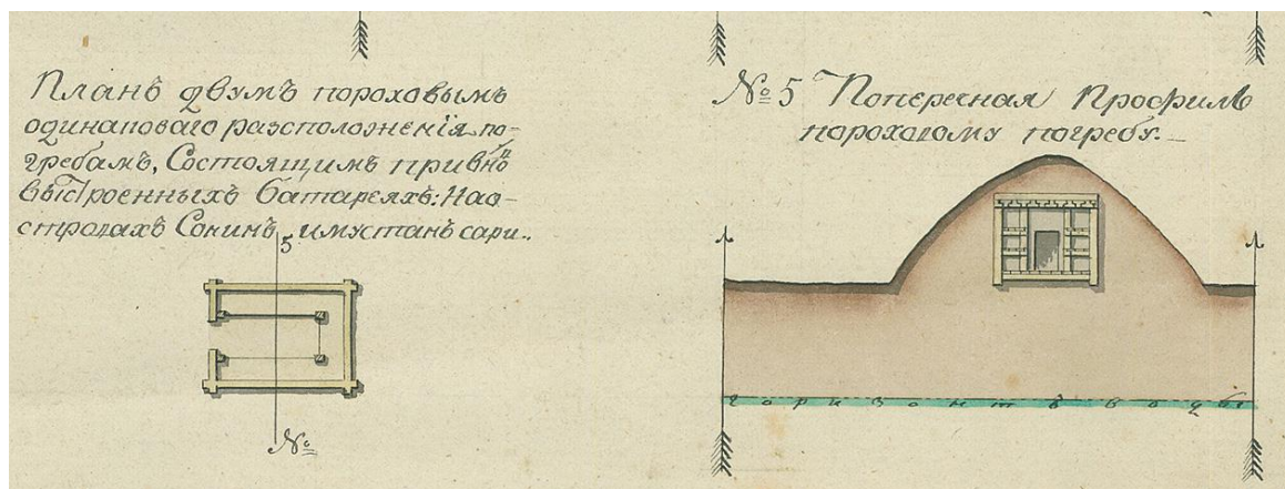
Пороховой снарядный погребъ при батарее Суонионсари. Фрагмент генплана. 1808 г. Источник: Национальный архив Финляндии.
