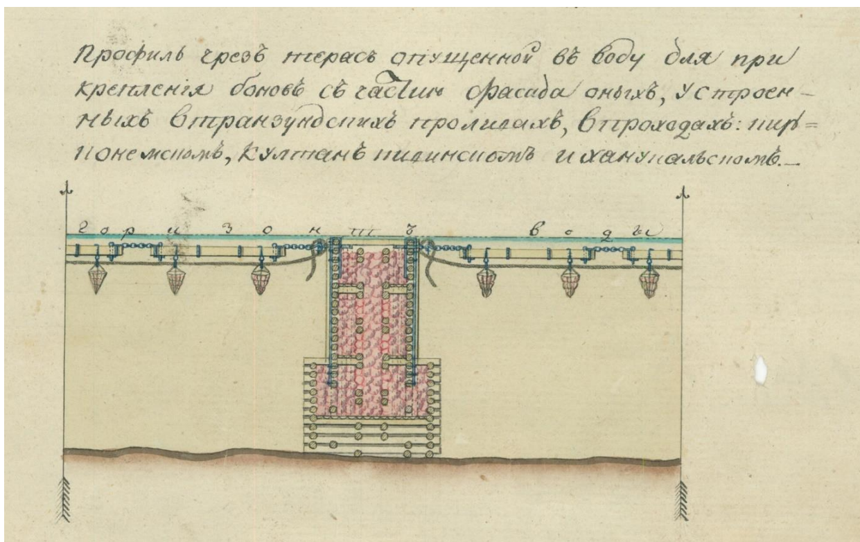
Конструкция бонъ, установленных в проливе между островами Суонионсари и Култанквисари. 1808 г. Источник: Национальный архив Финляндии.
