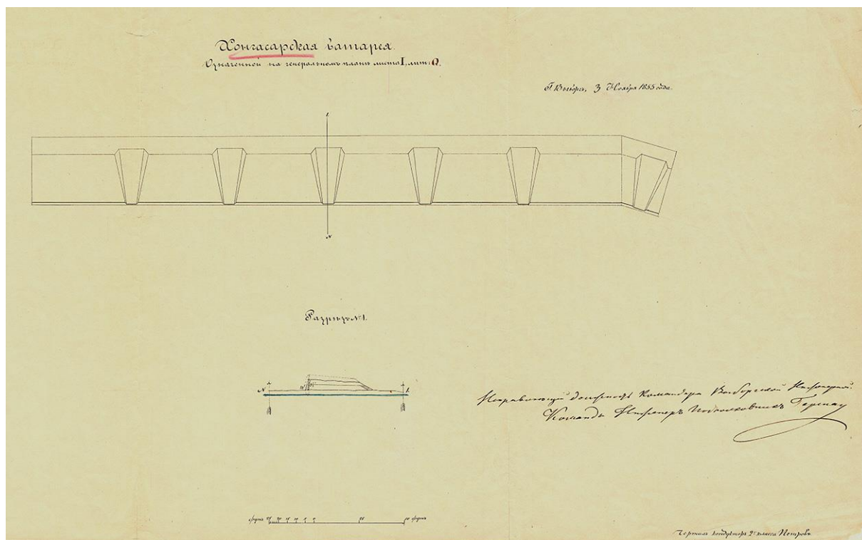
Генеральный план Хонгасарской батареи. 3 ноября 1855 г. Источник: цифровой фонд Национального архива Финляндии.
