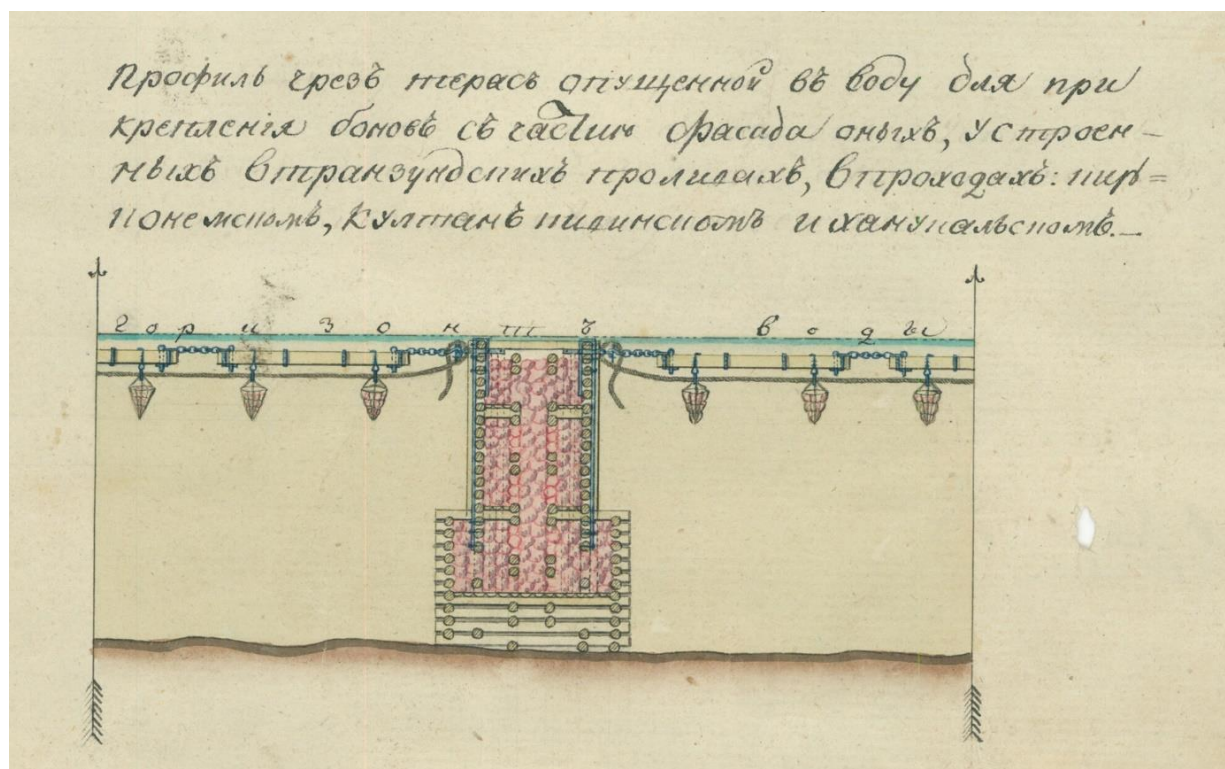
Конструкция подводного заграждения пролива (бона) у батареи Кирккониеми. Фрагмент генплана. 1808 г. Источник: цифровой фонд Национального архива Финляндии.
