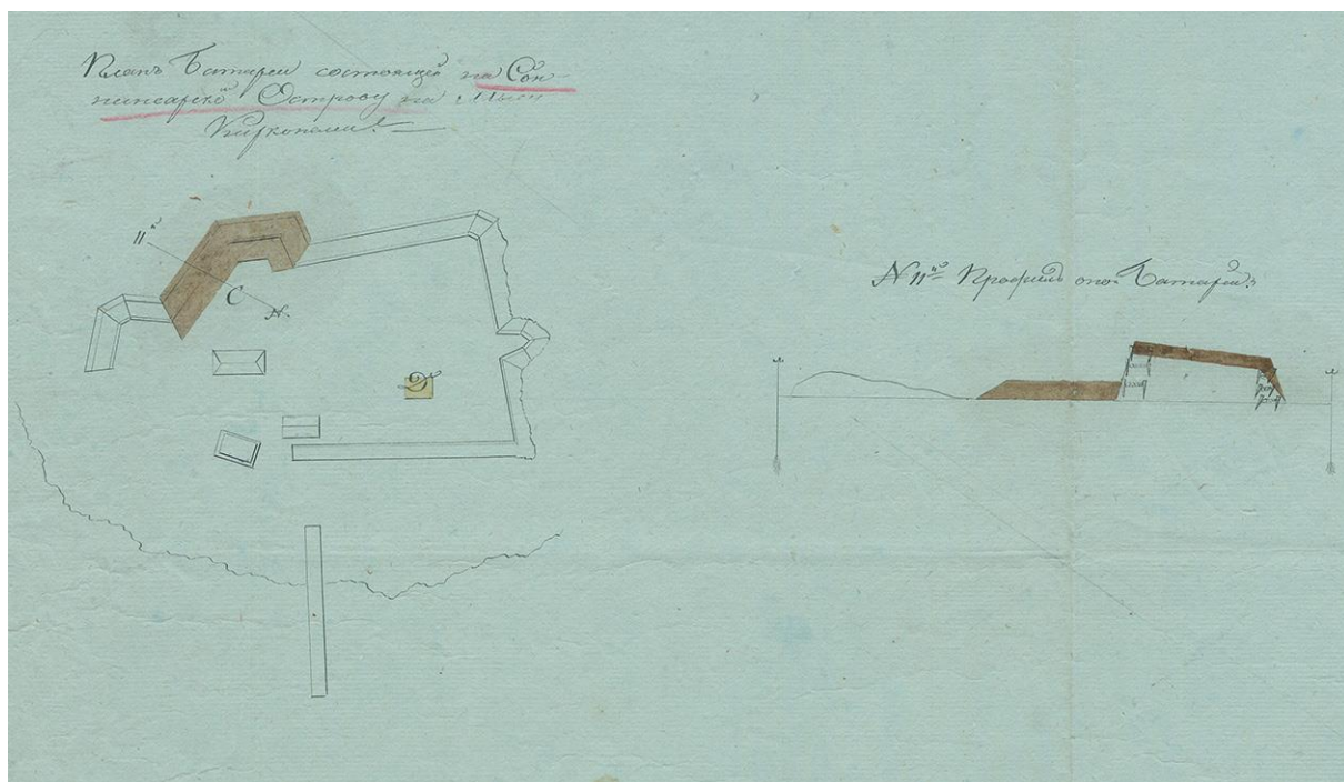
Ремонт редута Кирккониemi, разрушенного штормом. Генплан с показанием «перестроенного вновь» порохового погреба и поперечный разрез бруствера. 1811 г. Источник: цифровой фонд Национального архива Финляндии.
