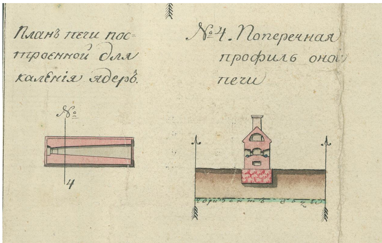
Проект печи для каления ядер на территории батареи. Фрагмент Генплана. 1808 г. Источник: цифровой фонд Национального архива Финляндии.
