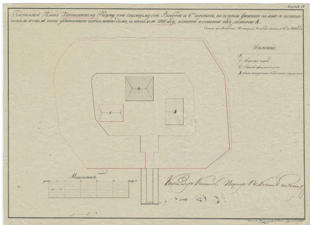
Генеральный план Ханкесарского редута, отстоящего от Выборга в 6 верстах, на острове финского залива с показанием вновь устроенного караульного дома, в прошлом 1821 году, который и означен под литерою А. 28 февраля 1823 года. Источник: цифровой фонд Национального архива Финляндии.
