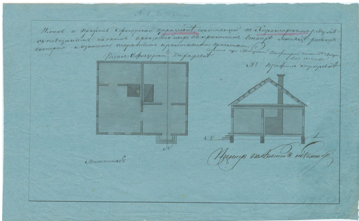
План и профиль офицерской караульни, состоящей в Ханкисарском редуте (...), 1822 год. Источник: цифровой фонд Национального архива Финляндии.
