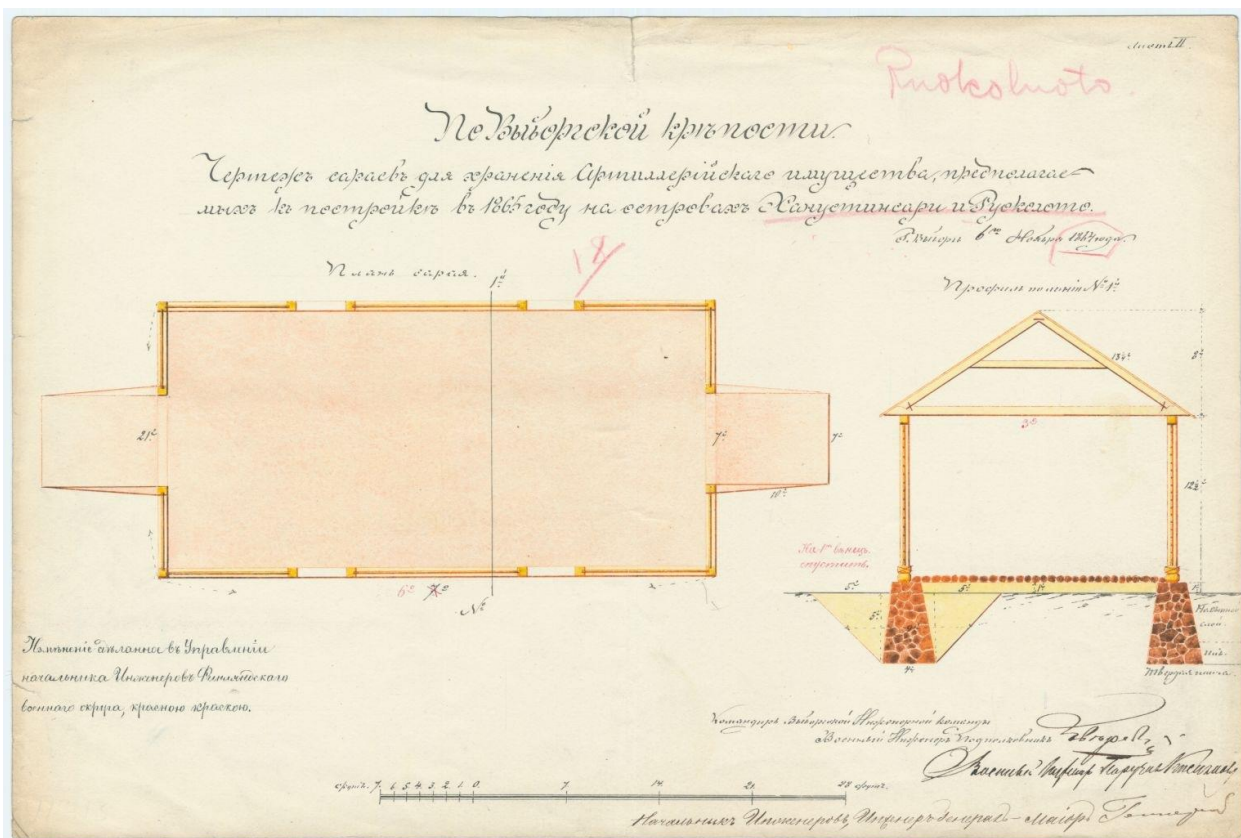
Чертеж сараев для хранения артиллерийского имущества, предполагаемый к постройке в 1865 году на островах Ханустинсари и Руоколотто. г.Выборг, 6 ноября 1864 г. Источник: Цифровой фонд Национального архива Финляндии.
