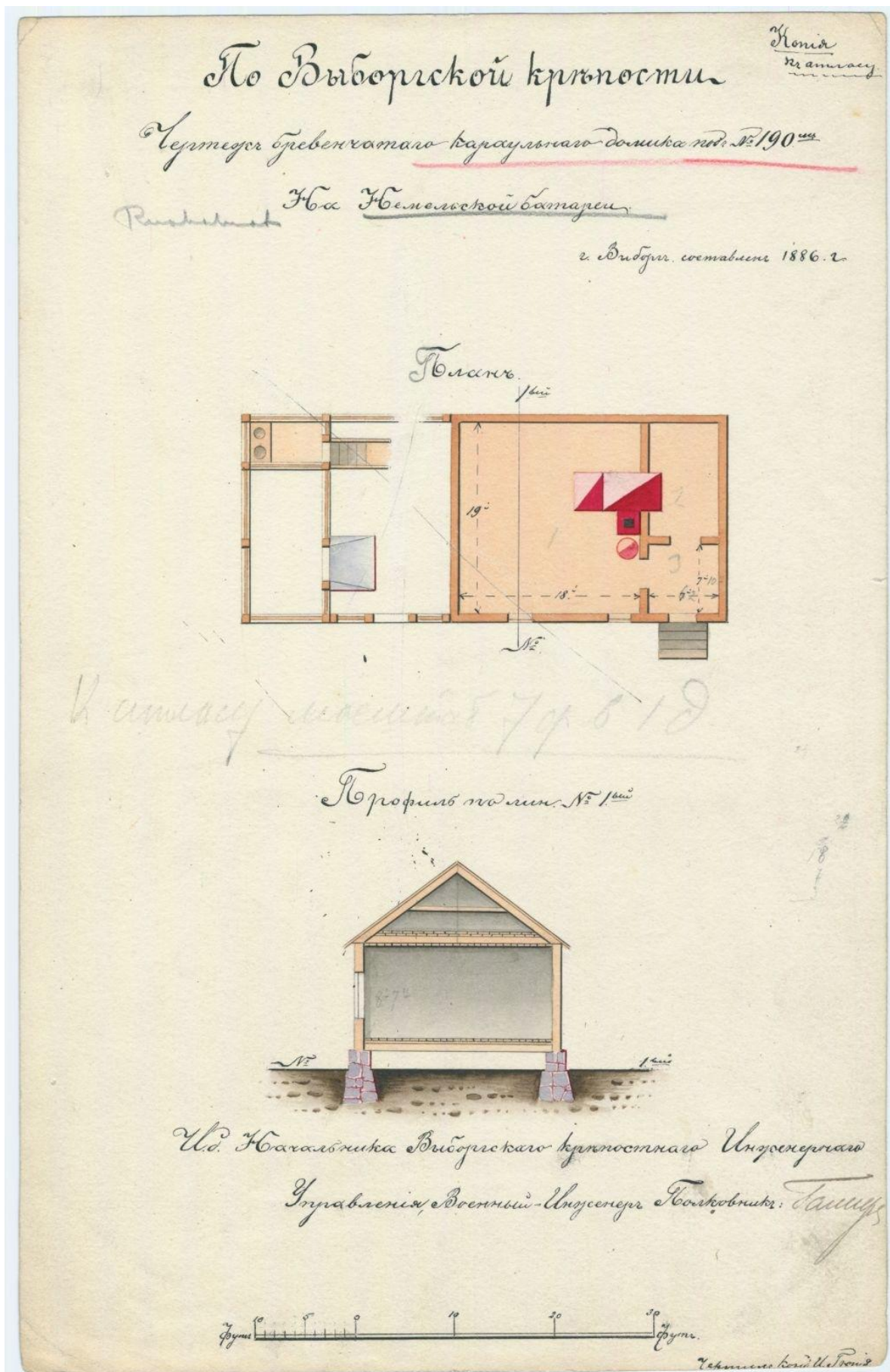
Чертеж бревенчатого караульного домика на Ниемльской батарее. 1886 г. Источник: Цифровой фонд Национального архива Финляндии.
