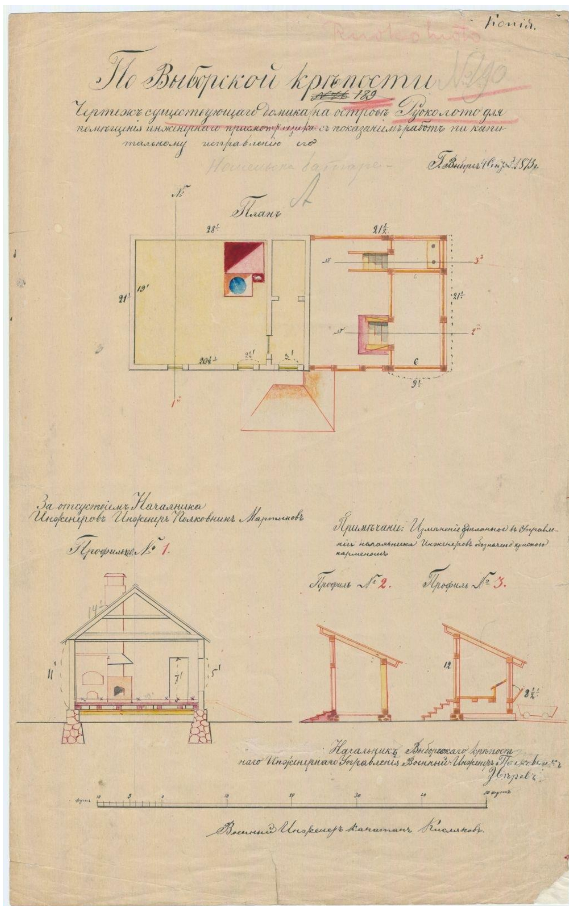
Чертежъ существующаго караульнаго домика на островѣ Руколомѣ для помещенія инженернаго присмотрщика. 1873 г. Источник: Цифровой фонд Национального архива Финляндии.
