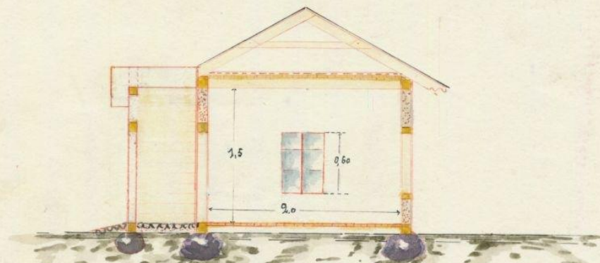
Разрѣзъ по № 1
