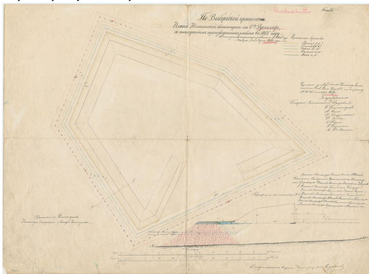
План Ниемльской батареи с показанием проведенных работ в 1865 г. г. Выборг, 31 июля 1868 г.
