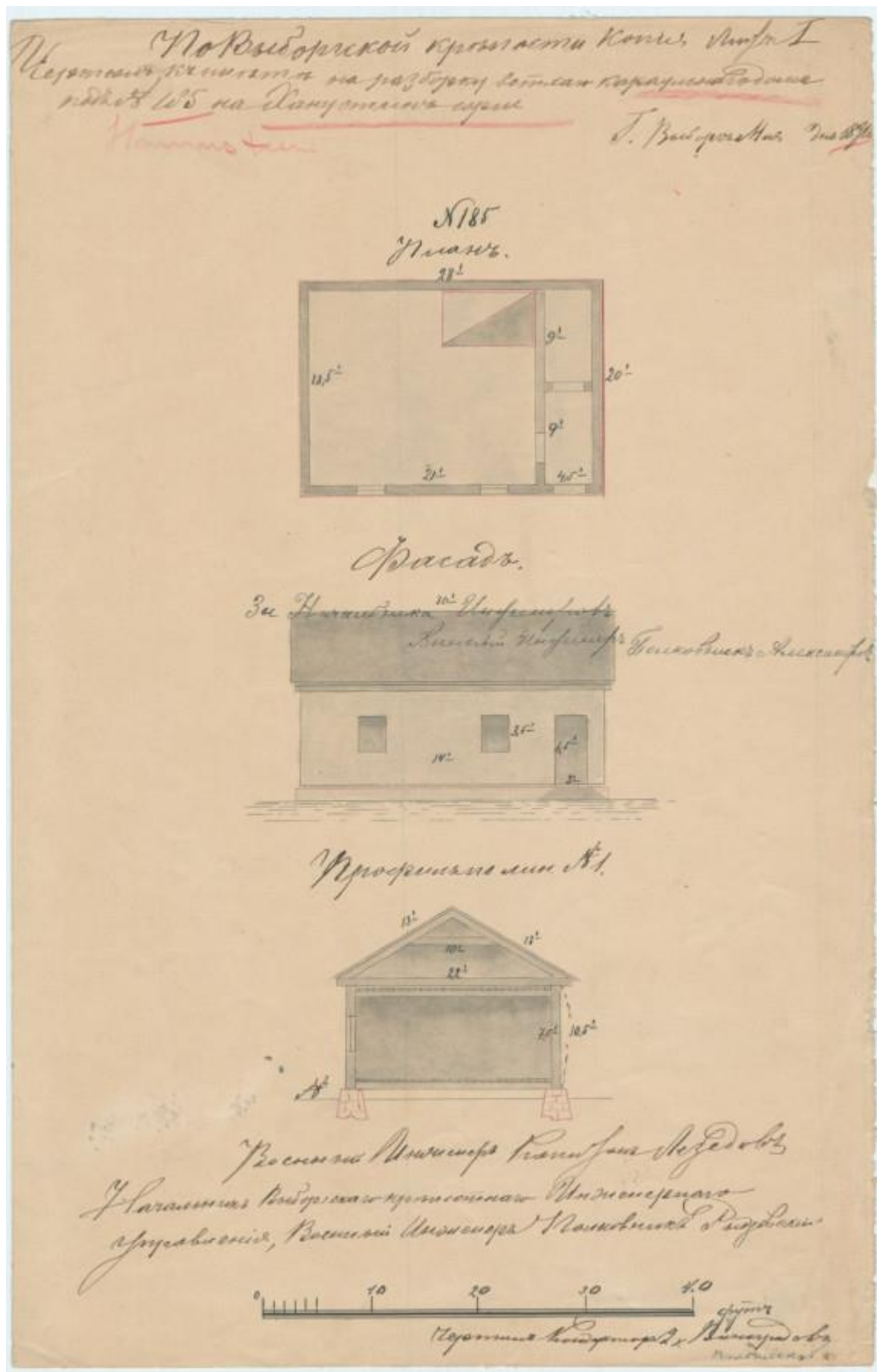
Чертеж на разборку ветхого караульного дома под №185 на Ханнустиенсаари. г. Выборг, 1891 г. Источник: Цифровой фонд Национального архива Финляндии.
