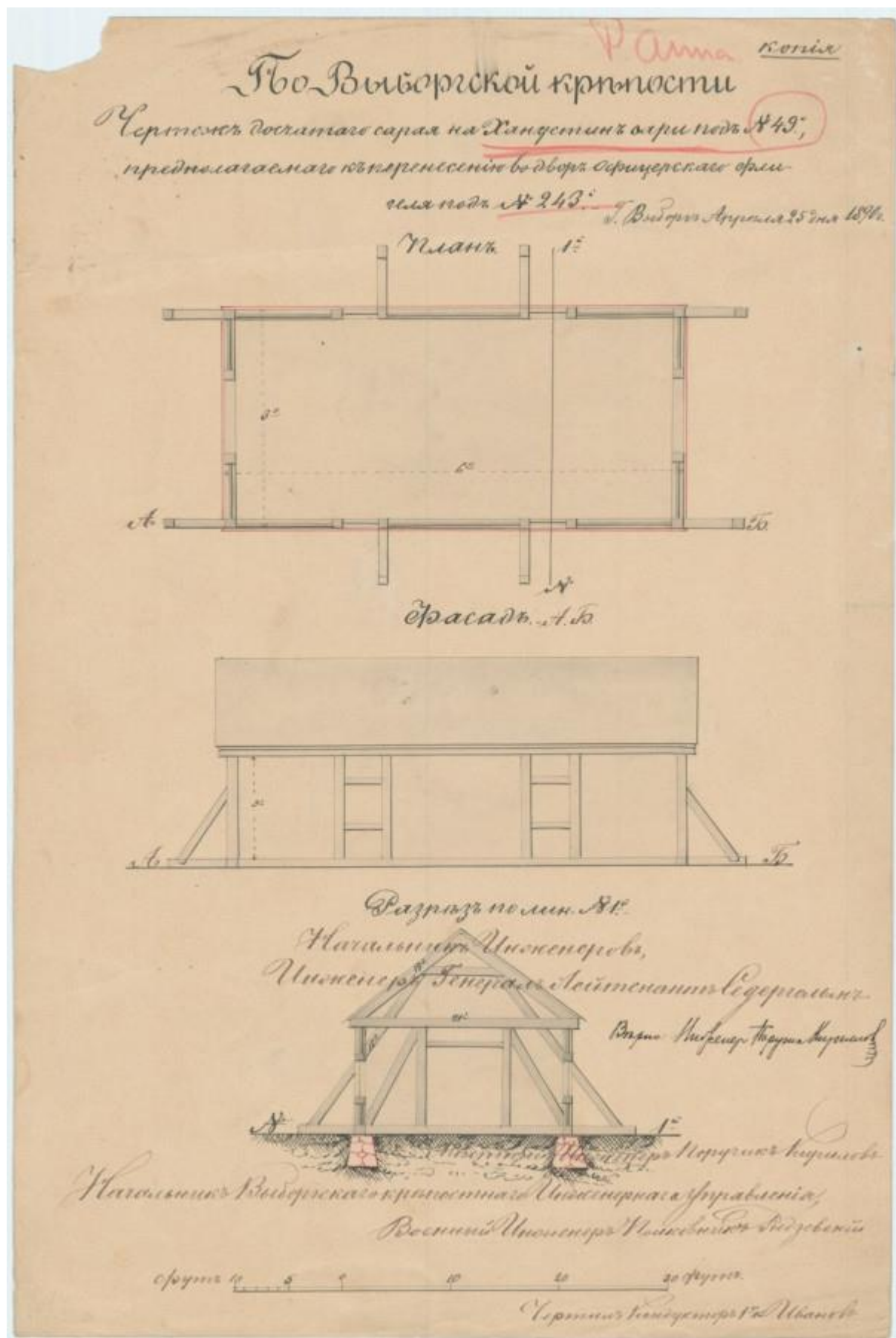
Чертеж дощатого сарая №185 на Ханнустиенсаари под №49 предлагаемого к перенесению во двор офицерского флигеля №243. г. Выборг, 1891 г. Источник: Цифровой фонд Национального архива Финляндии.
