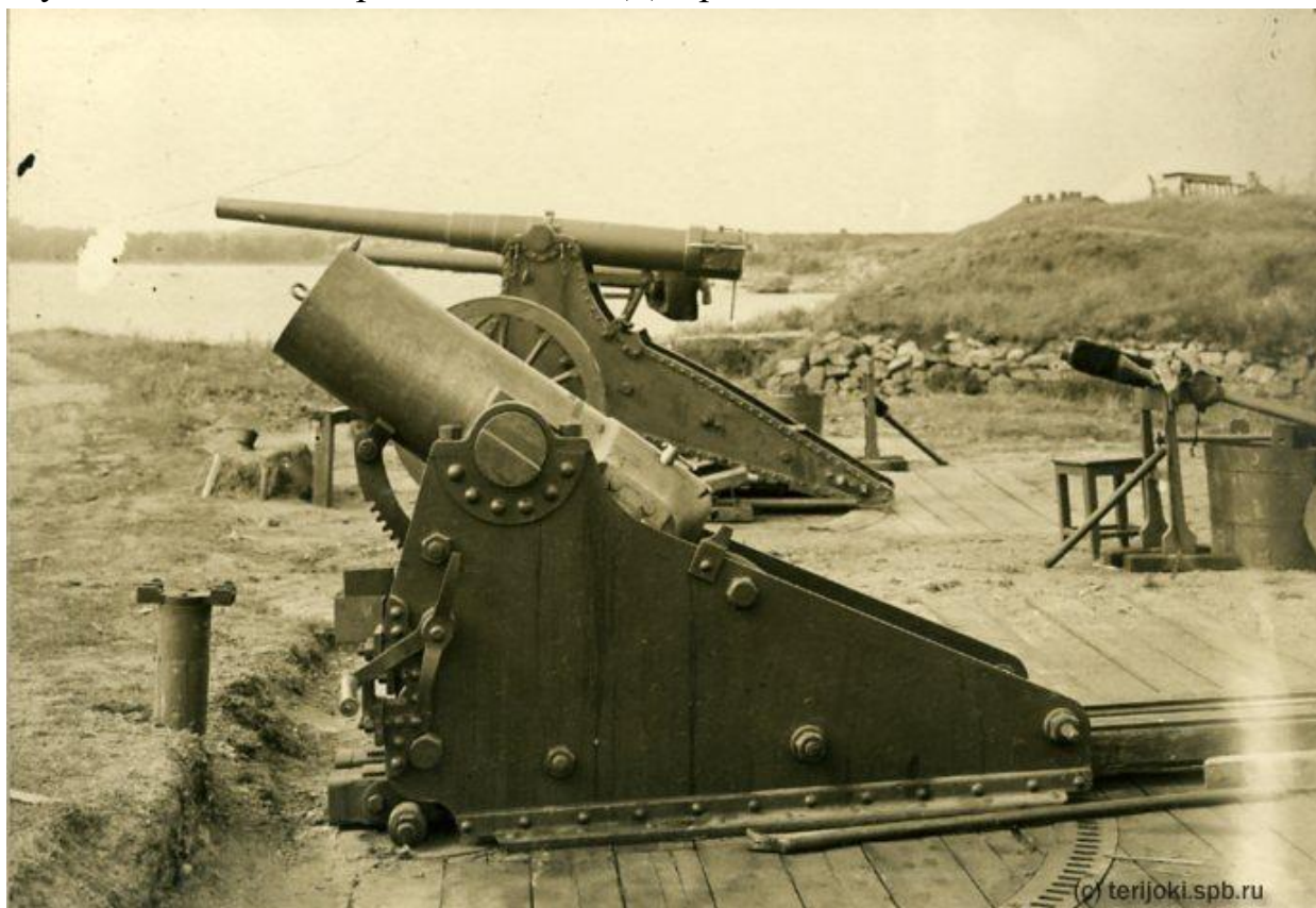
Пример размещения орудий на островных батареях. Источник: www.terijoki.spb.ru
