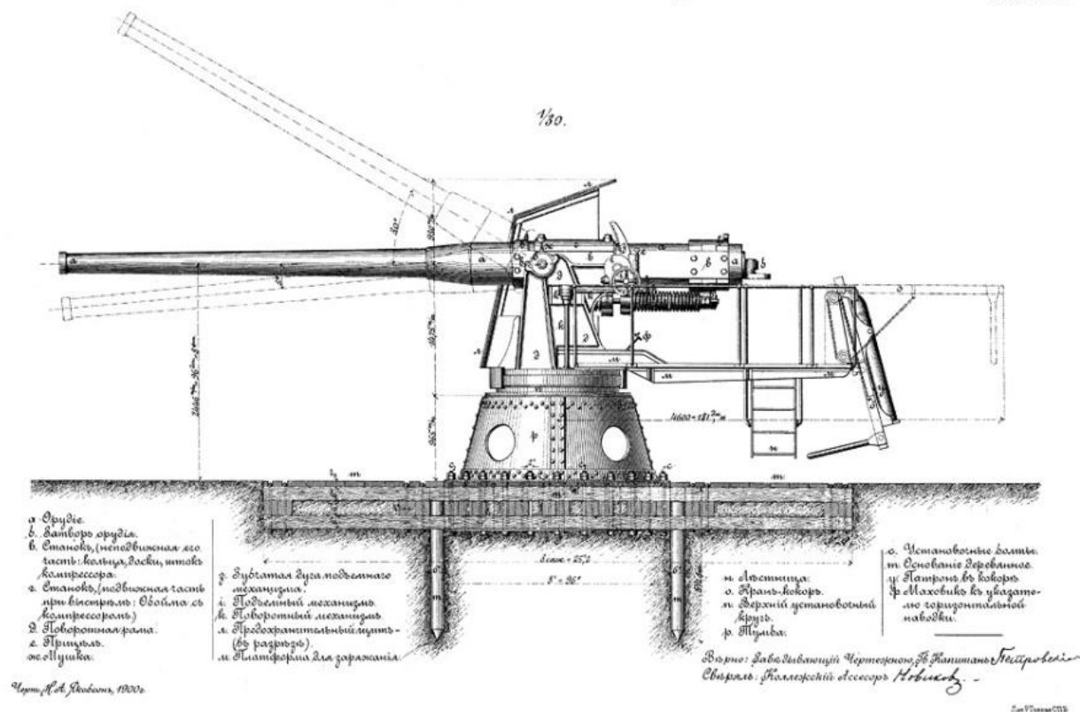
Общий вид установки Канэ. 1900 г.
