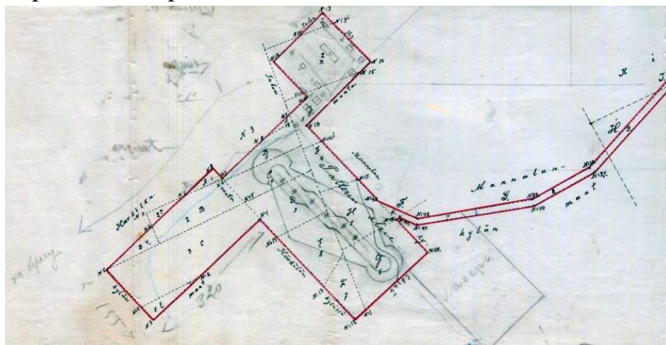
Схема расположения береговой батареи Хяркяля Источник: https://www.glebychevo.narod.ru/vihor.html
