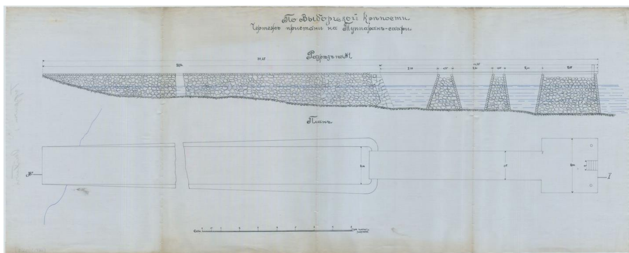
Чертеж пристани на Гуппурансаари. Документ из цифровых фондов Национального архива Финляндии.
