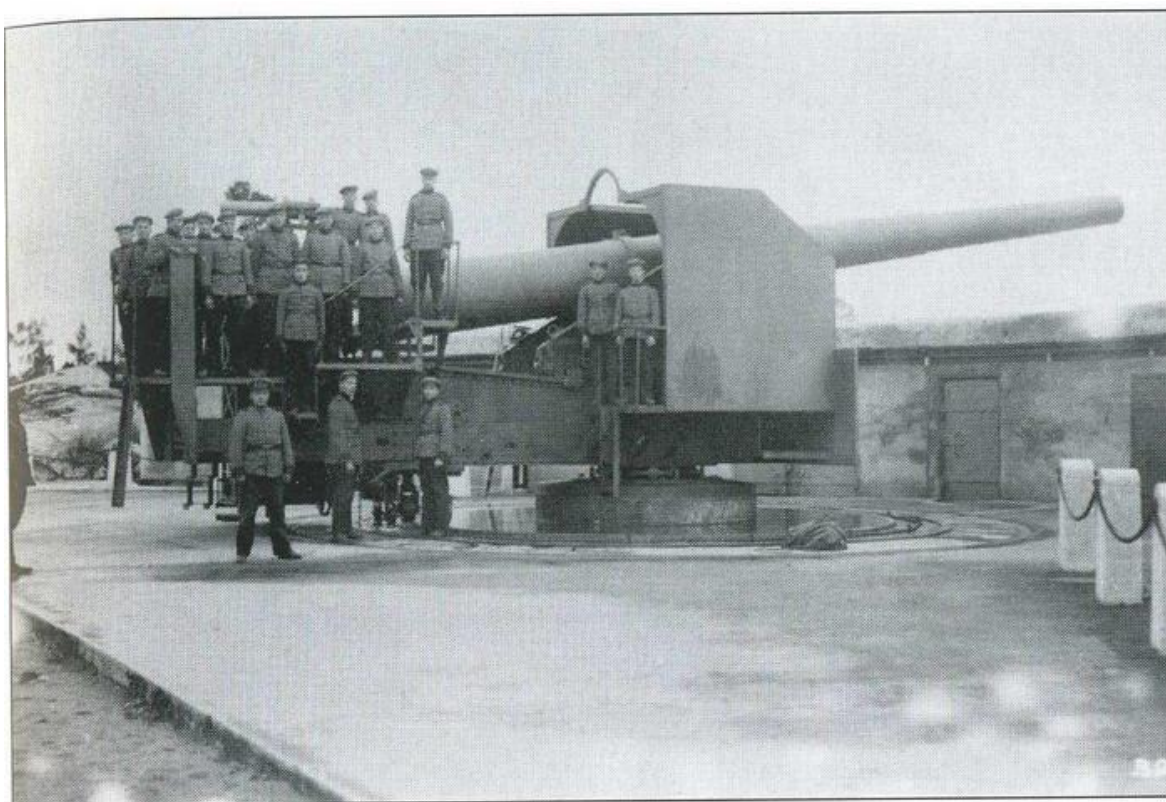
254-мм пушка на станке Дурляхера, переделанная финнами Пушка на станке Дурляхера калибра 254 мм. Источник: www.zwezet.turbina.ru
