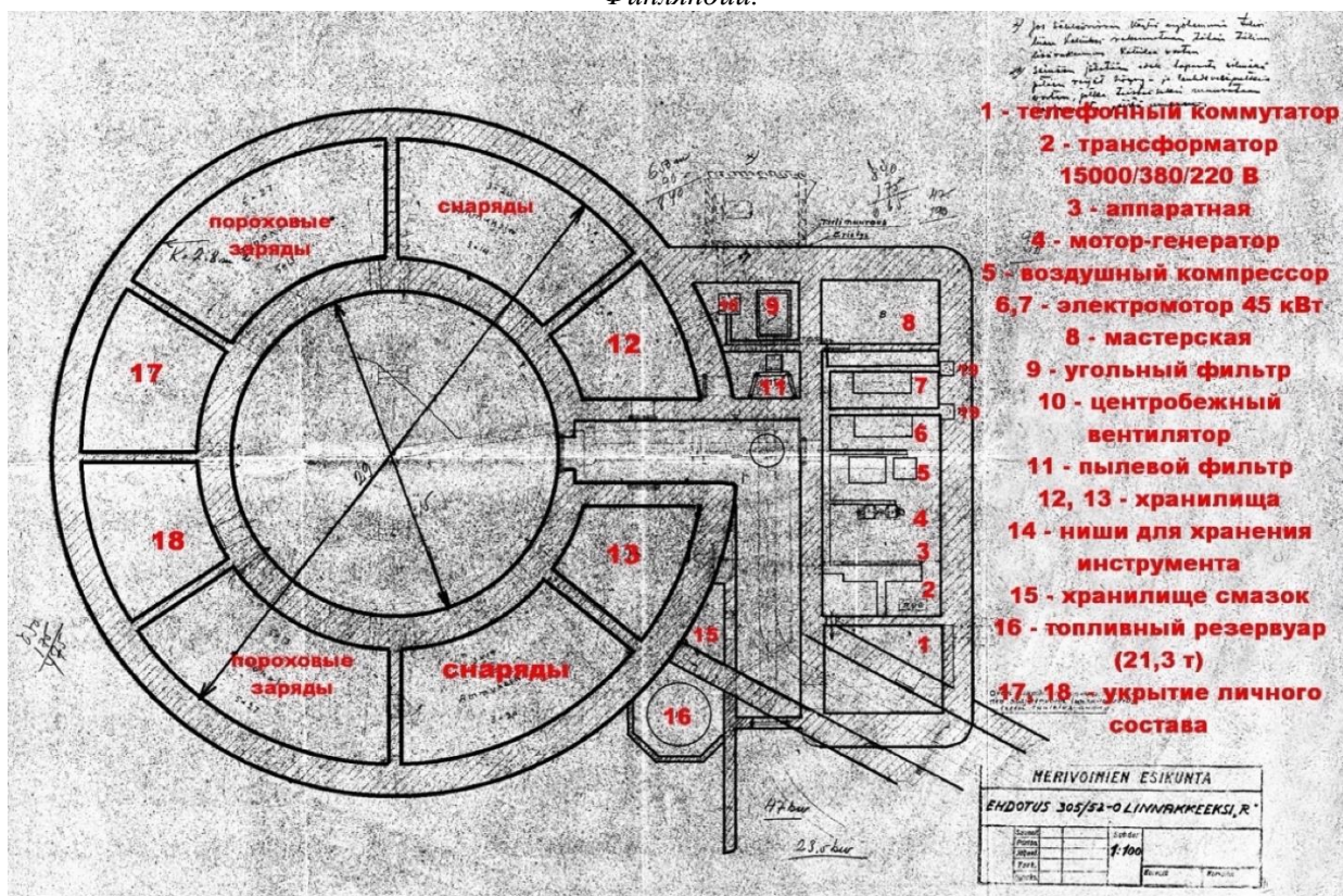
Схема орудийной установки. Источник: https://lenobl-travel.livejournal.com/538072.html
