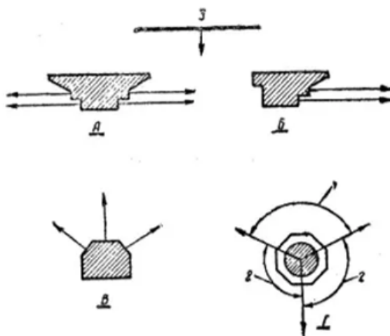
Рис. 2. Виды казематированных огневых фортификационных сооружений: А — огневое сооружение флангового действия — капонир; Б — огневое сооружение флангового действия — полукaponир; В — огневое сооружение фронтального действия; Г — огневое сооружение с круговым обстрелом: 1 — основной сектор огня, 2 — дополнительный сектор огня, 3 — противник
