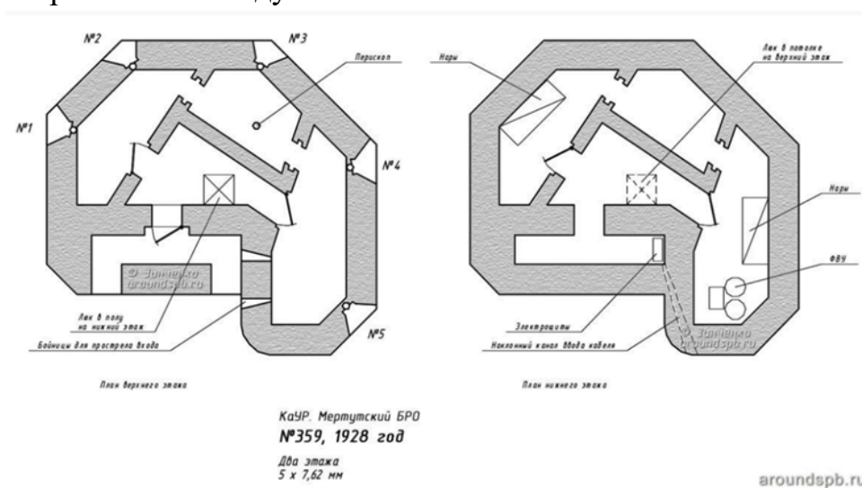
Полтажний план ДОТа №359
