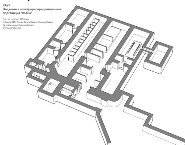
Подземная электроподстанция в Лемболово. 1933 г. Источник: https://www.aroundspb.ru
